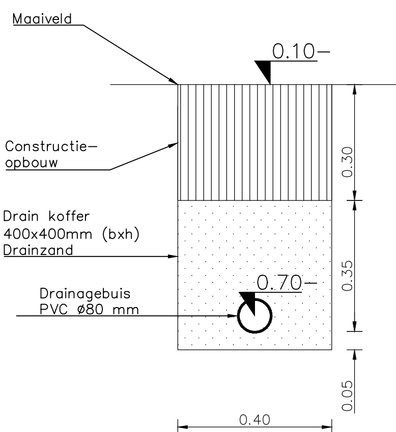
PRINCIPE DOORSNEDE DRAINKOFFER
