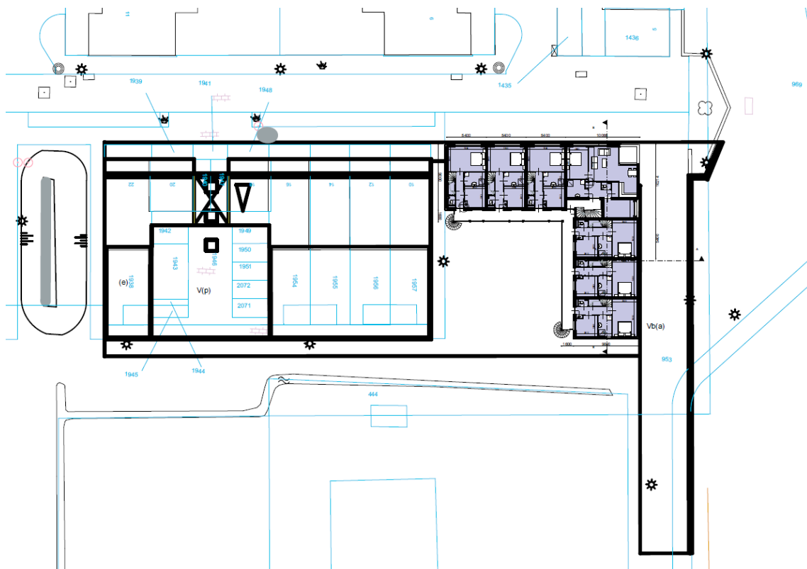
Afbeelding 2.2: inpassing in stedenbouwkundige opzet De Villa
