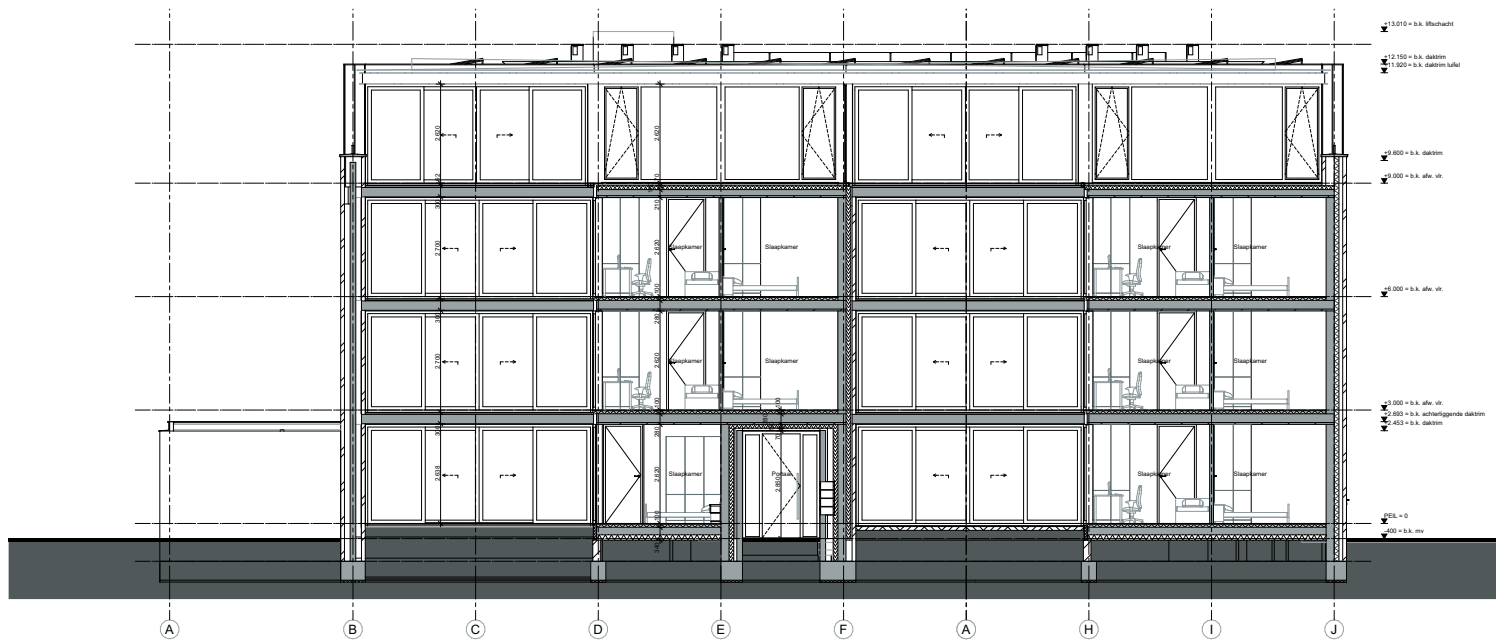
DOORSNEDE D-D
