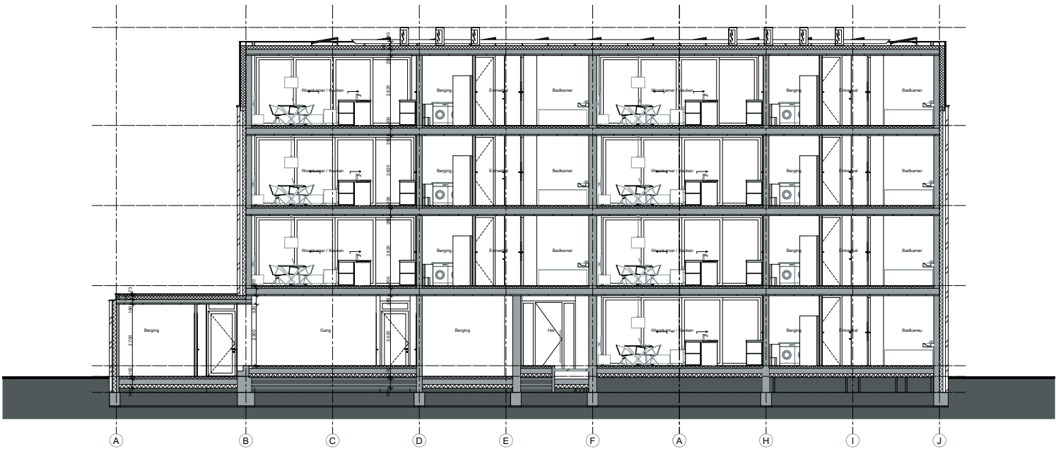
DOORSNEDE F-F
