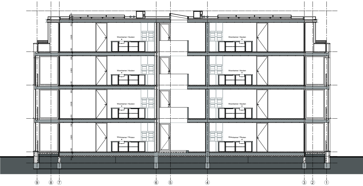
DOORSNEDE C-C
