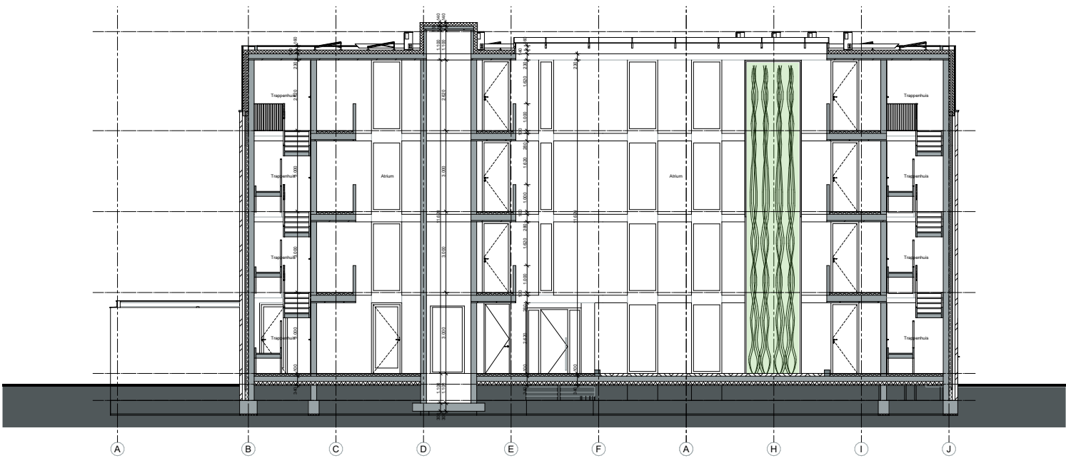
DOORSNEDE E-E
