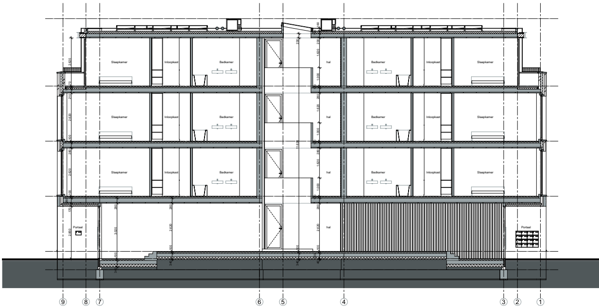
DOORSNEDE B-B
