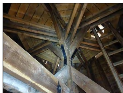
Figuur 18. Constructie toren, zicht op tweede platform met koekoek ramen.
