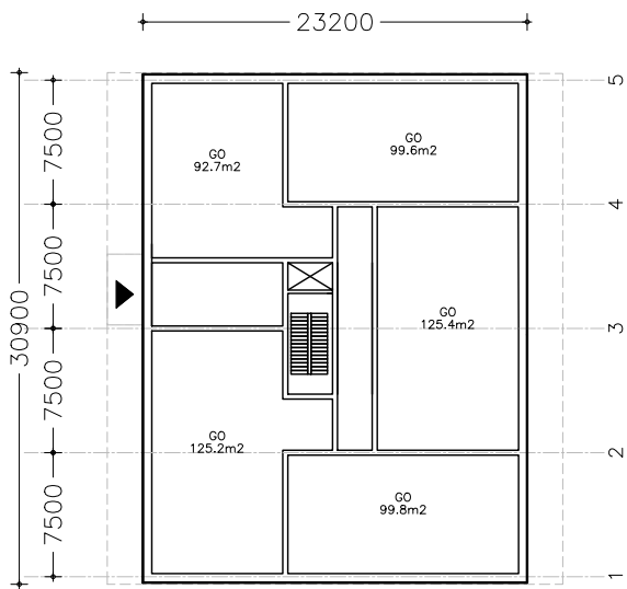
begane grond
