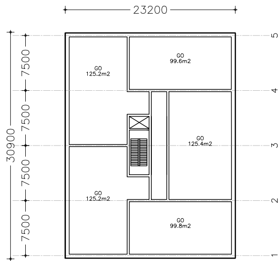
verdieping 1
