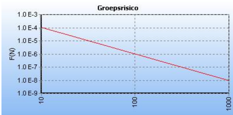
5.2 Figuur 5.2 FN curve voor Z-511-01 van N.V. Nederlandse Gasunie voor de kilometer tussen stationing 8510.00 en stationing 9510.00
