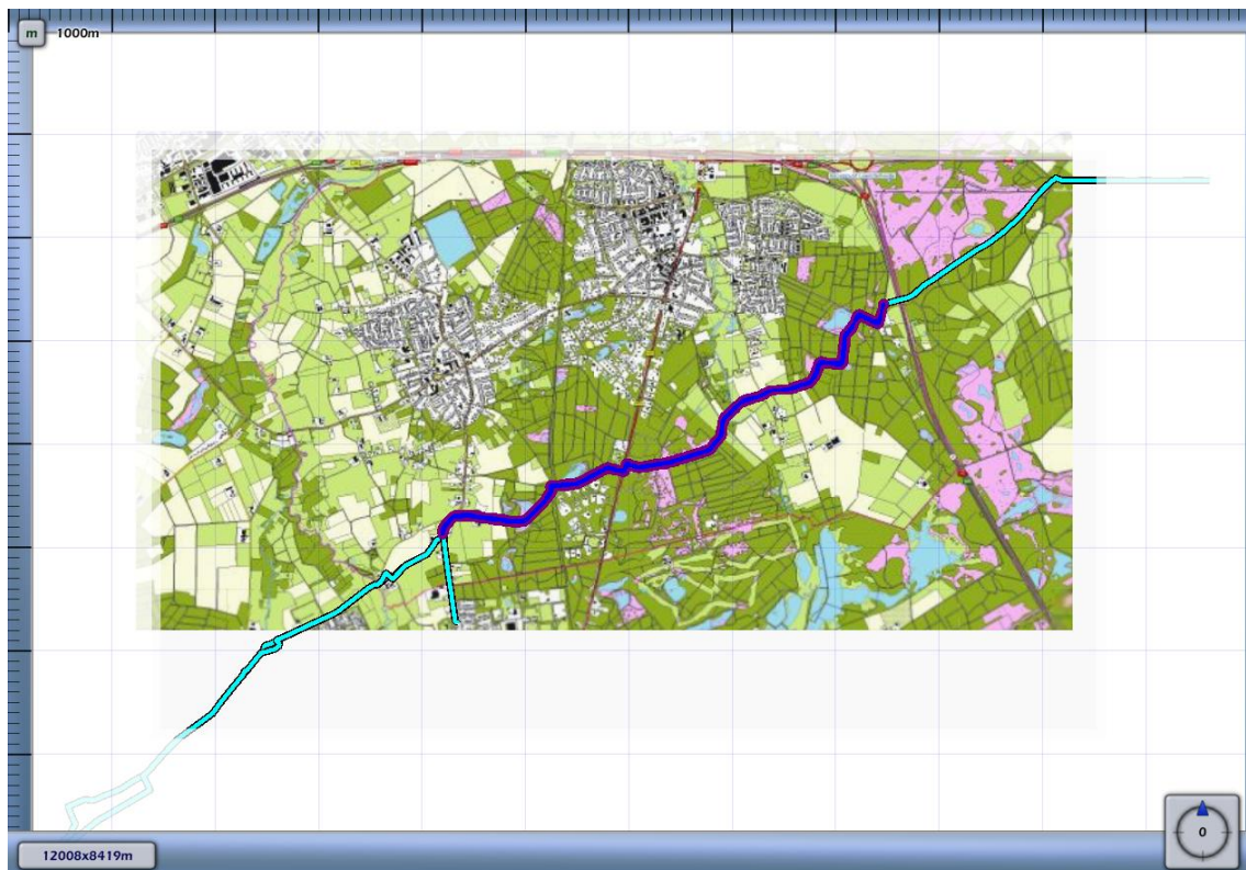
3.1 Figuur 3.1 Plaatsgebonden risico voor Z-511-06 van N.V. Nederlandse Gasunie
