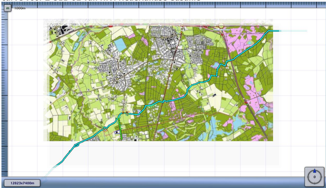
Figuur 4.3 Kilometer leiding behorende bij de maximale overschrijding van de FN-curve voor Z-511-02 van N.V. Nederlandse Gasunie
