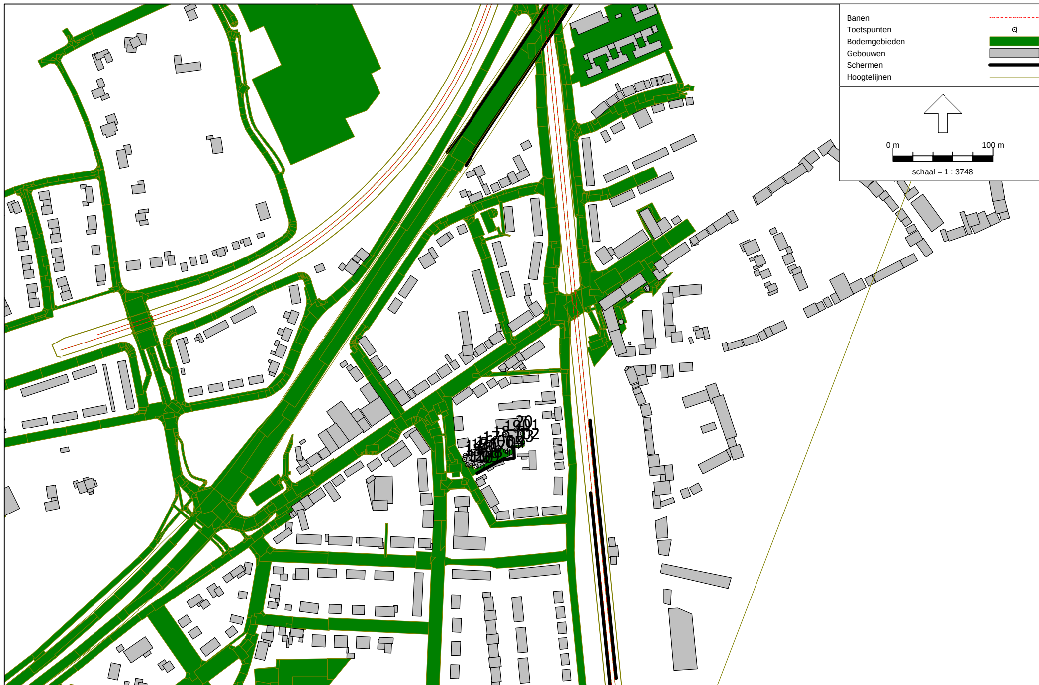
Figuur II-2 Overzicht rekenmodel railverkeer
