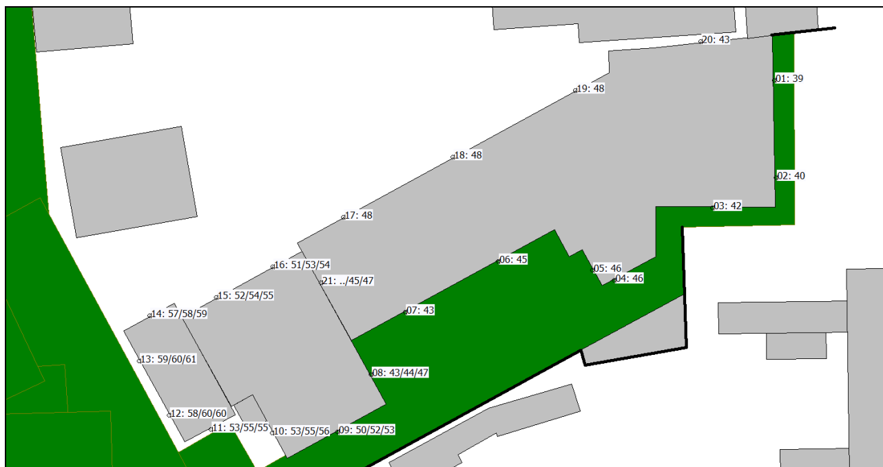
Figuur 4.3: Geluidbelasting t.g.v. wegverkeer op alle omliggende wegen (inclusief 30 km/uur wegen) (excl. aftrek art. 110g Wgh)
