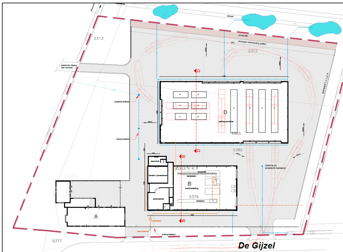
Weergave nieuwe situatie erfindeling en routes vrachtverkeer
