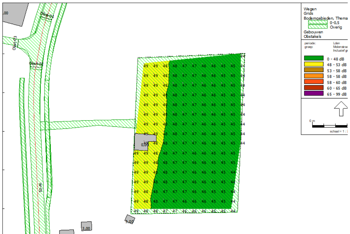
Figuur 3: Geluidcontour Molenstraat (incl. aftrek art. 110g Wgh) Berekende geluidbelastingen op een hoogte van 7,5 meter
