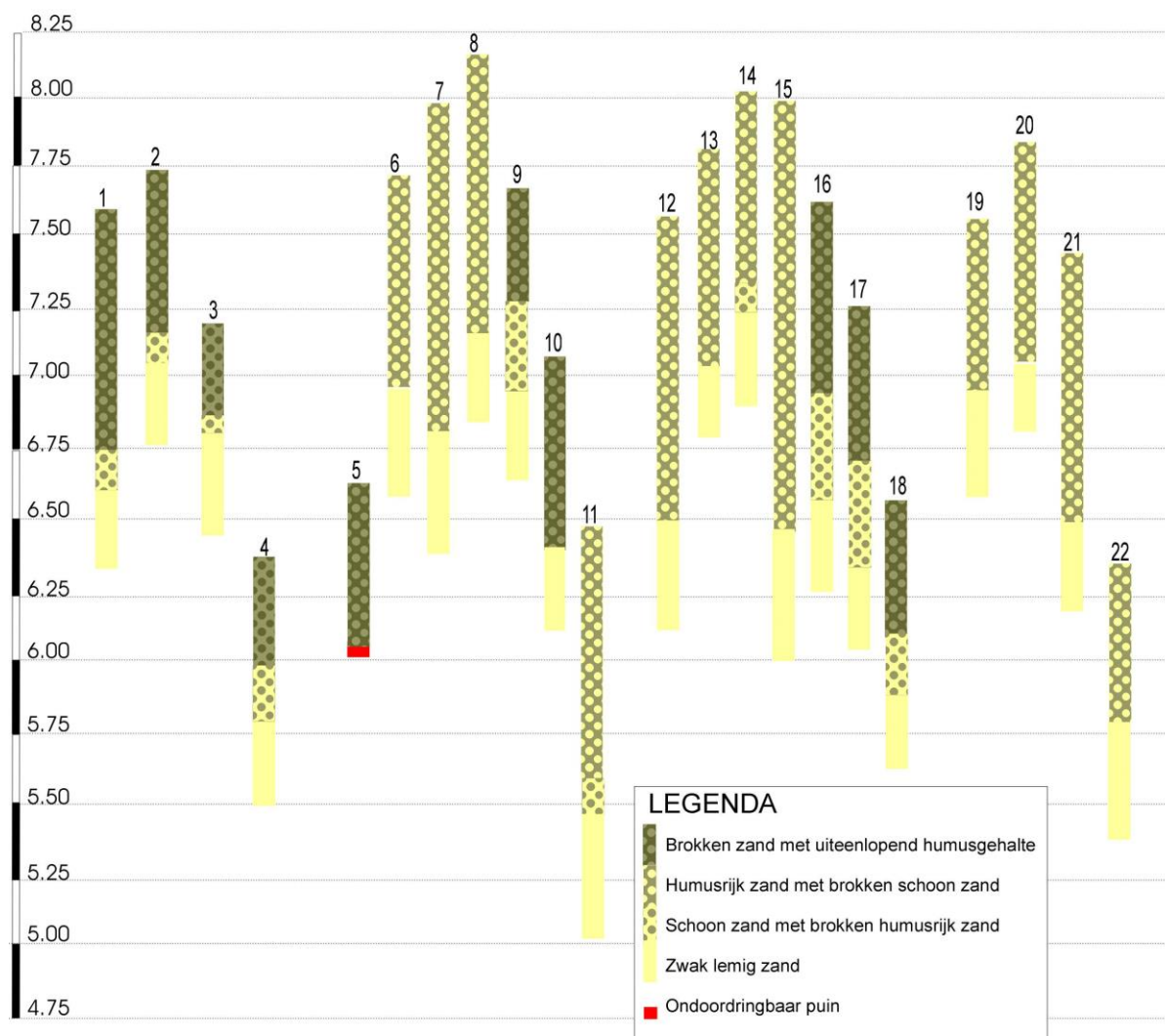
Figuur 37: Boorprofielen
