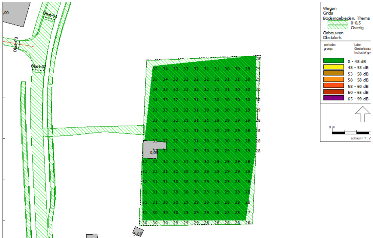
Figuur 6: Geluidcontour Gestelstraat (incl. aftrek art. 110g Wgh) Berekende geluidbelastingen op een hoogte van 7,5 meter
