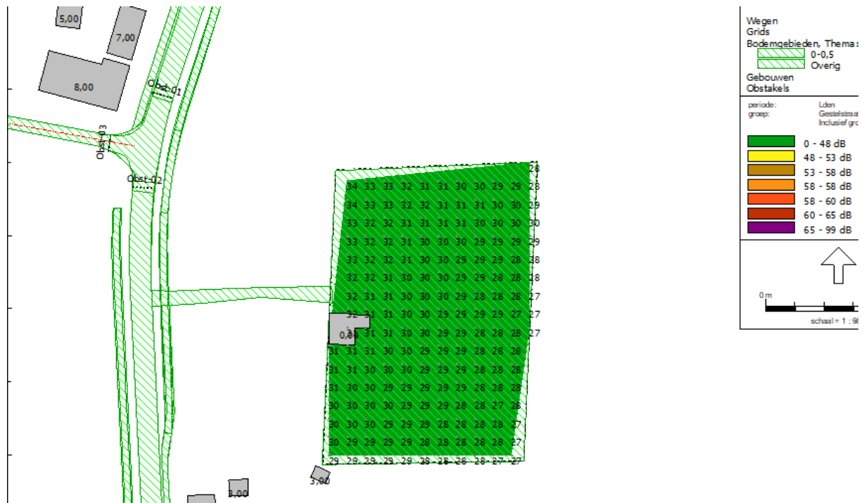
Figuur 5: Geluidcontour Gestelstraat (incl. aftrek art. 110g Wgh) Berekende geluidbelastingen op een hoogte van 4,5 meter
