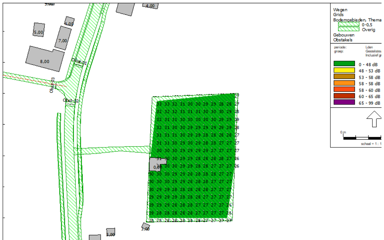
Figuur 4: Geluidcontour Gestelstraat (incl. aftrek art. 110g Wgh) Berekende geluidbelastingen op een hoogte van 1,5 meter
