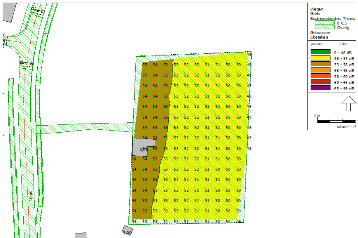
Figuur 7: Geluidcontour gecumuleerde geluidbelasting (excl. aftrek art. 110g Wgh) Berekende geluidbelastingen op een hoogte van 7,5 meter
