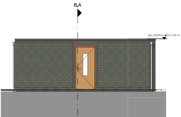
BERGING RECHTER ZIJGEVEL
