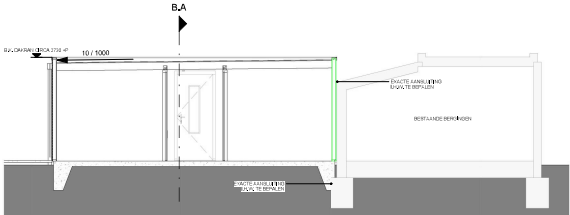
DOORSNEDE B.1
