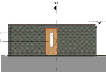
BERGING LINKER ZIJGEVEL
