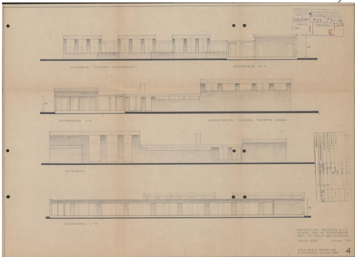
Gevel en doorsneden definitieve ontwerp (Bron: Regionaal Historisch Centrum Eindhoven, archiefnummer 10847)
