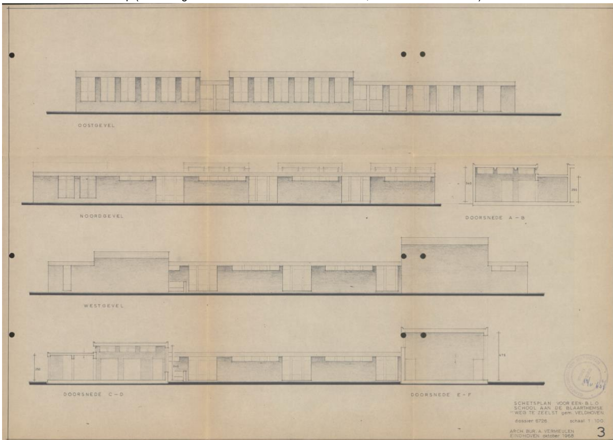
Gevel en doorsneden definitieve ontwerp (Bron: Regionaal Historisch Centrum Eindhoven, archiefnummer 10847)
