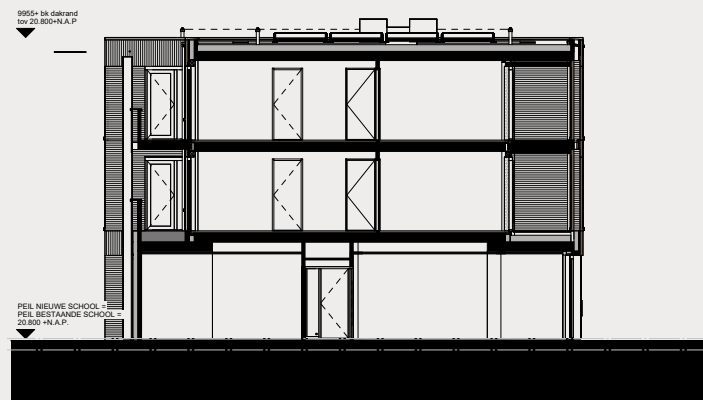
Doorsnede A
