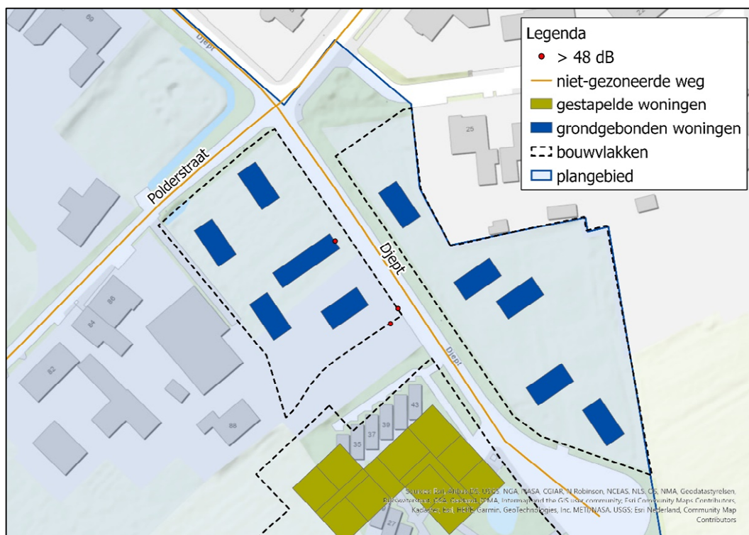
Figuur 4.4 Toetspunten met een geluidbelasting hoger dan 48 dB als gevolg van de niet-gezoneerde wegen in en nabij het plangebied.
