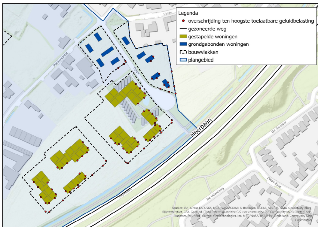
Figuur 4.1 Toetspunten met een overschrijding van de ten hoogste toelaatbare geluidbelasting als gevolg van verkeer op de Heerbaan.
