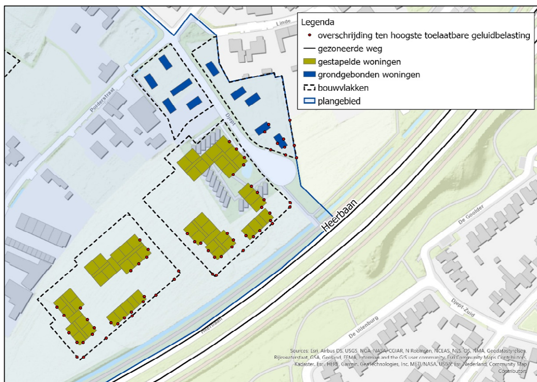
Figuur 4.6 Toetspunten met een overschrijding van de ten hoogste toelaatbare geluidbelasting als gevolg van verkeer op de Heerbaan na toepassing van de voorgestelde bronmaatregel.
