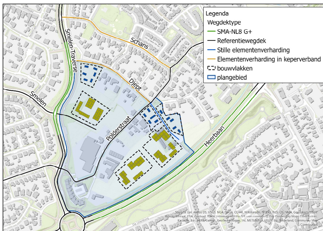
Figuur 4.5: Schematische weergave van de ligging van de besproken bronmaatregelen.
