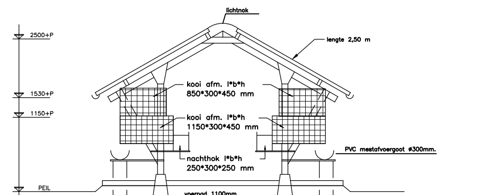
Doorsnede A1-A1 (sheds 7 t/m 14) SCHAAL 1:50 BB 94-02-013
