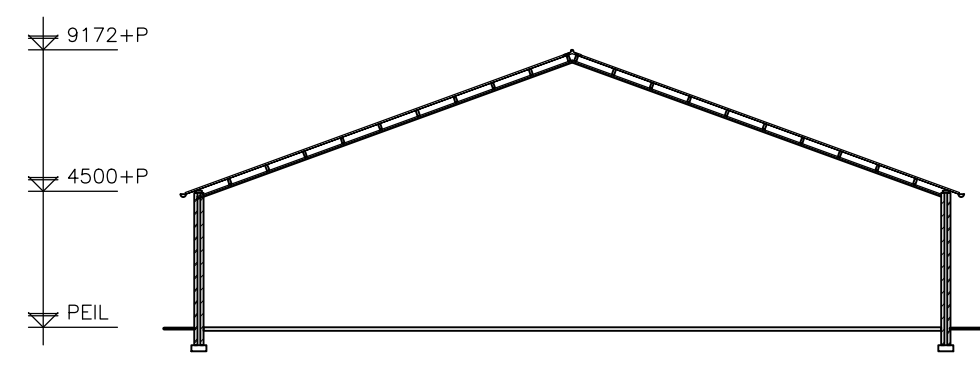
Doorsnede D-D
