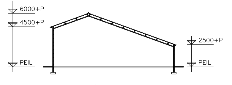
Doorsnede C-C
