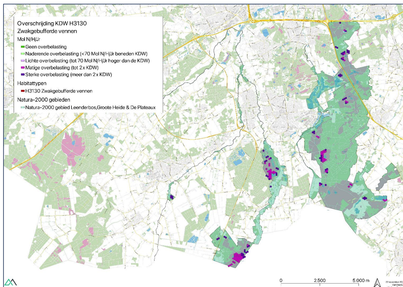
Figuur 5-5 Verspreiding en mate van overschrijding van de KDW van het habitattype H3130 Zwakgebufferde vennen in het Natura 2000-gebied Leenderbos, Groote Heide & De Plateaux (Bron: AERIUS Monitor, versie 2025).
