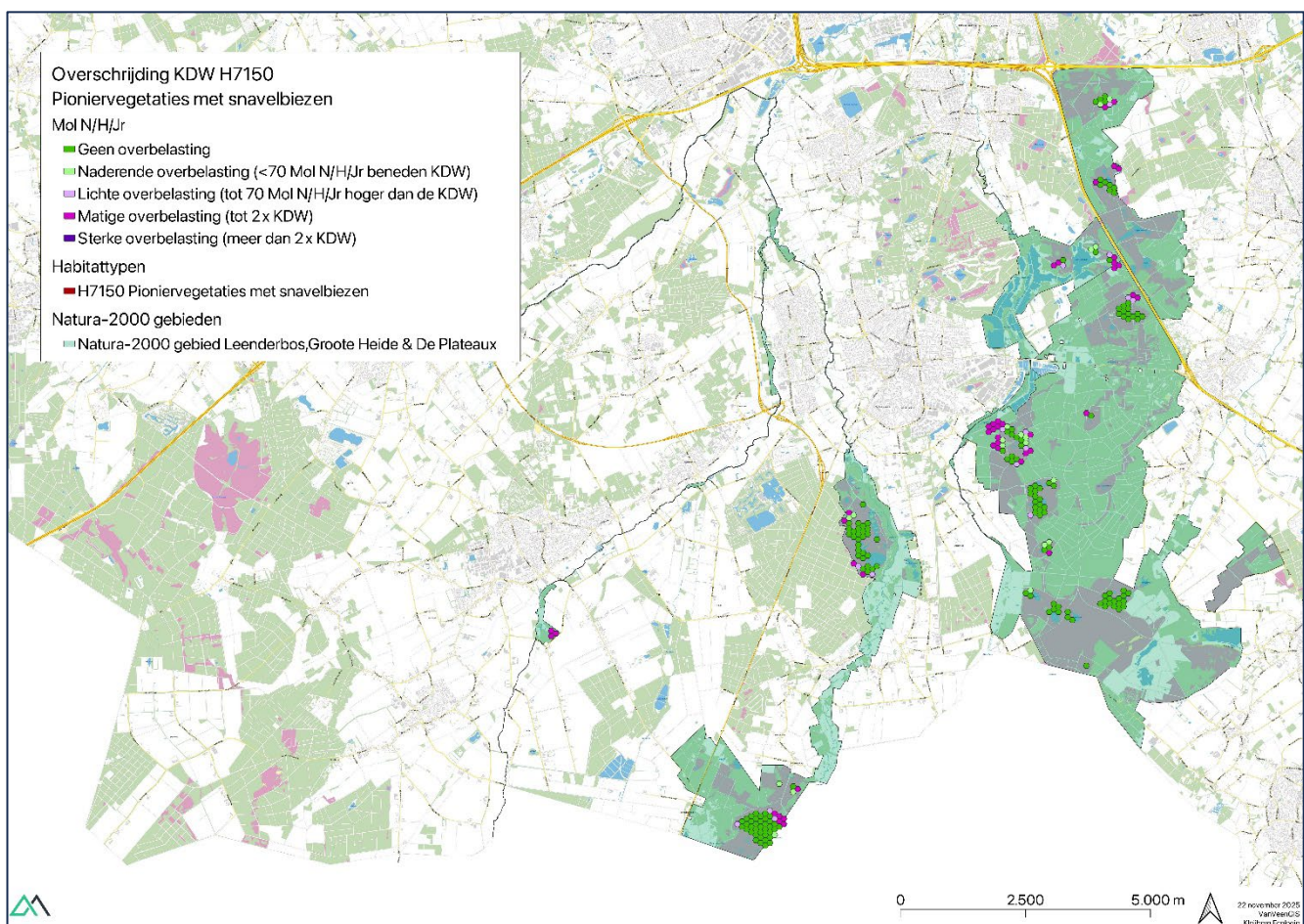
Figuur 5-9 Verspreiding en mate van overschrijding van de KDW van het habitatype H7150 Pioniervegaties met snavelbiezen in het Natura 2000-gebied Leenderbos, Groote Heide & De Plateaux (Bron: AERIUS Monitor, versie 2025).
