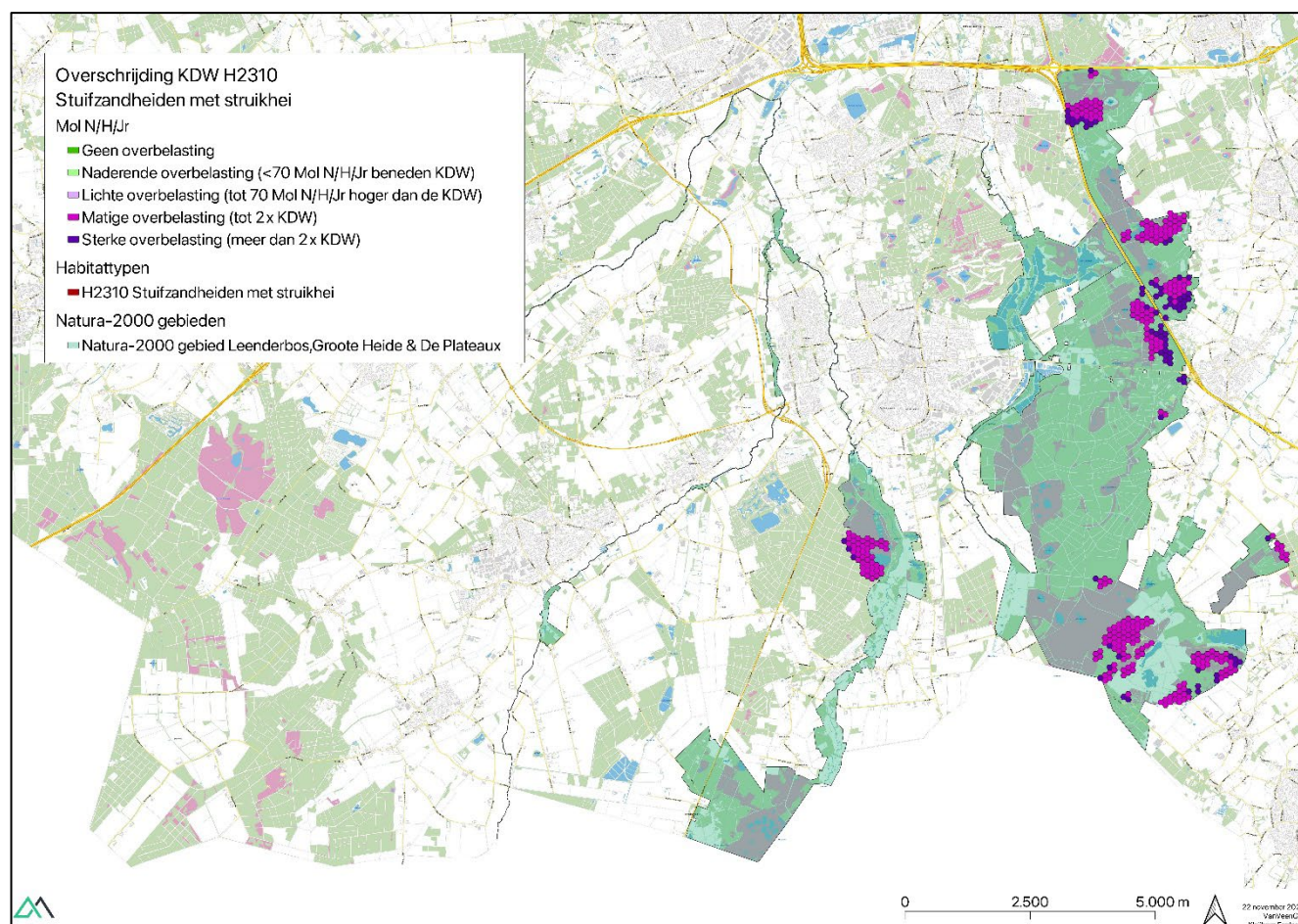
Figuur 5-4 Verspreiding en mate van overschrijding KDW van het habitattype H2310 Stuifzandheiden met struikhei in het Natura 2000-gebied Leenderbos, Groote Heide & De Plateaux (Bron: AERIUS Monitor, versie 2025).
