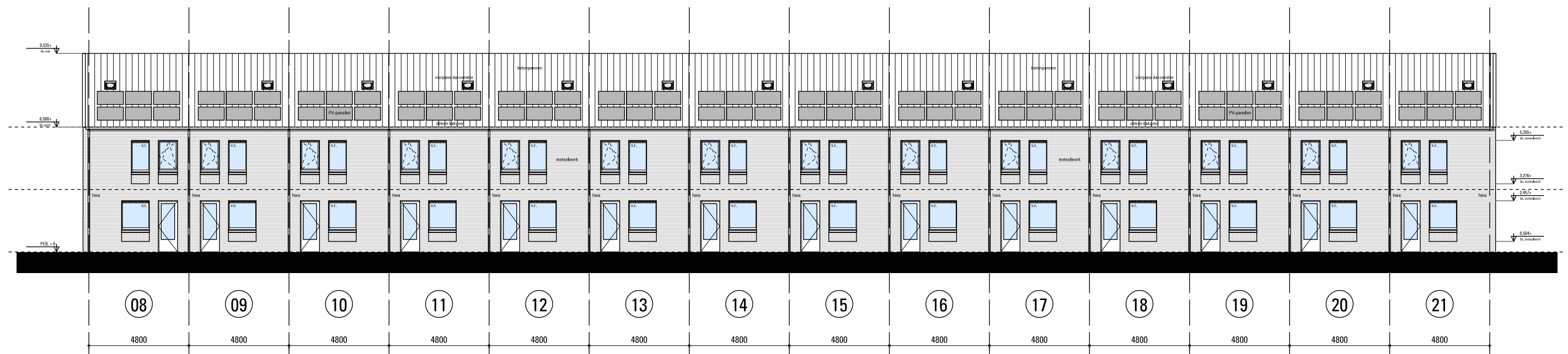
ACHTERGEVEL blok 2
