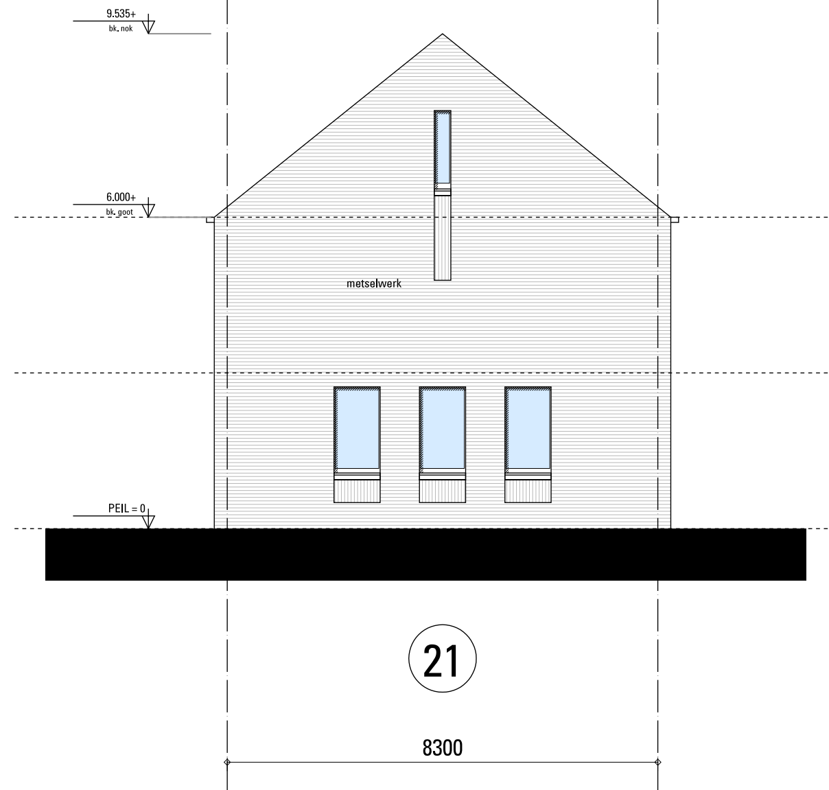
LINKER ZIJGEVEL
