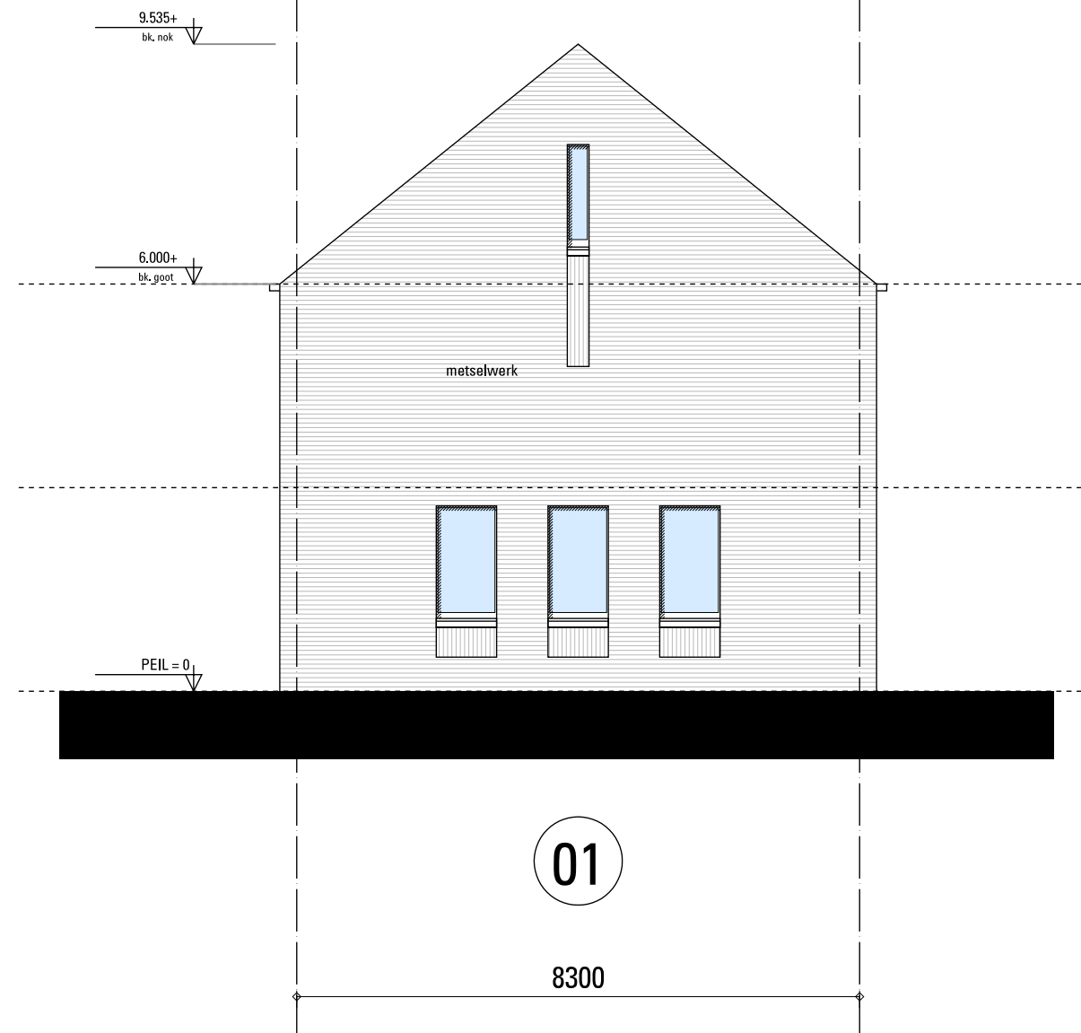
RECHTER ZIJGEVEL
