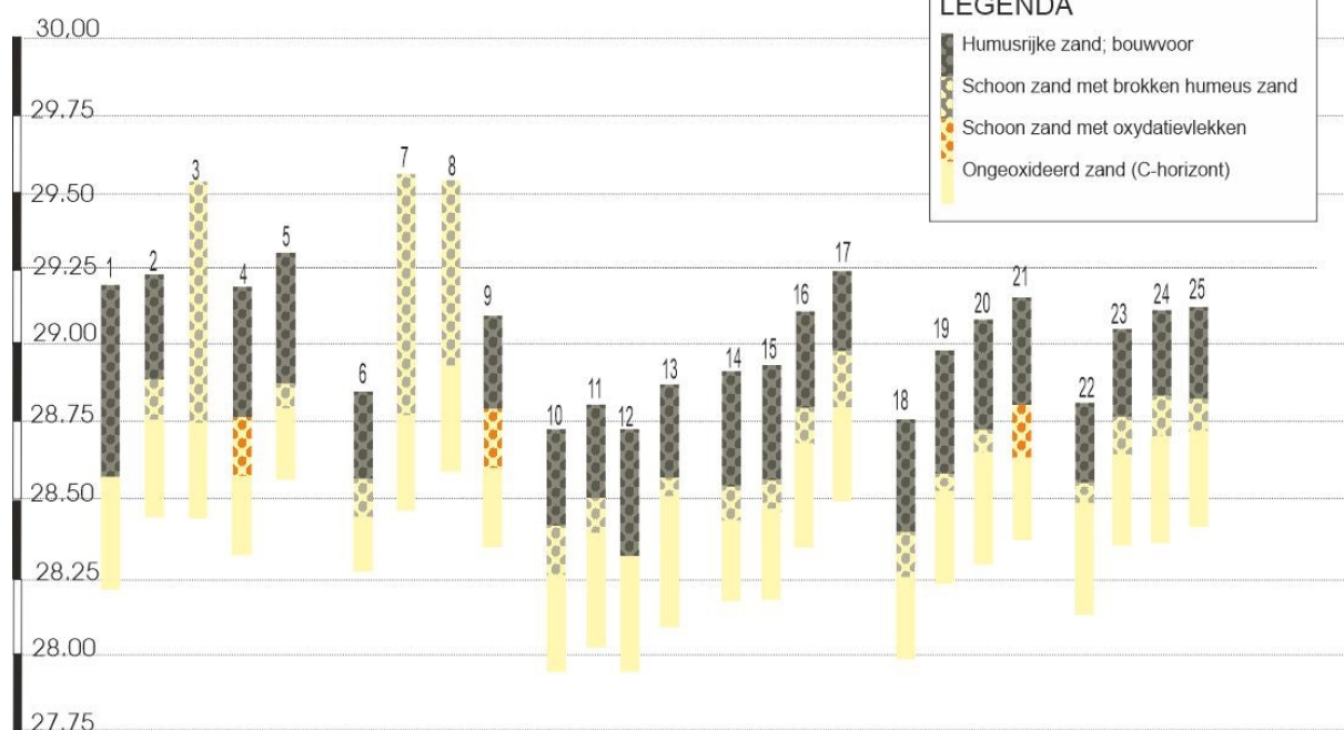
Figuur 26: Boorprofielen
