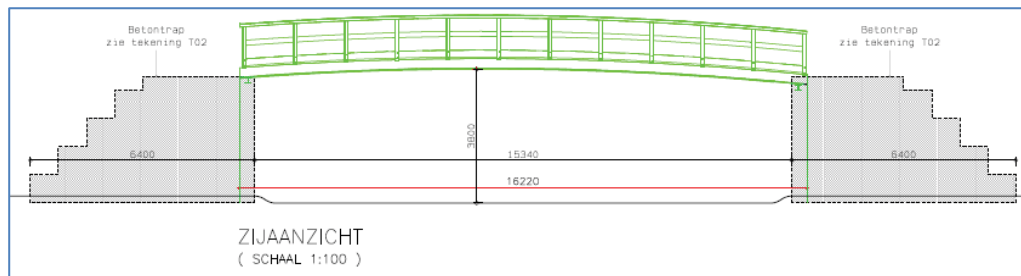
Figuur. Zijaanzicht loopbrug, Wouter Margry Architecten.
