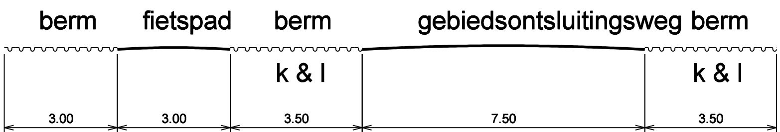
Dwarsprofiel 2
