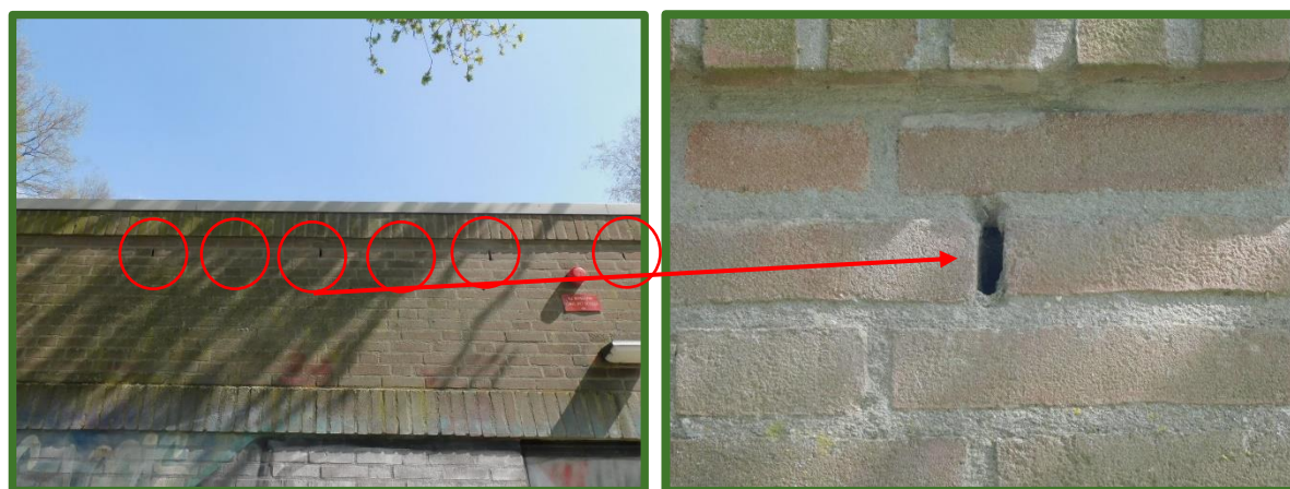
Overzicht muur transformatorhuisje met open stootvoegen
