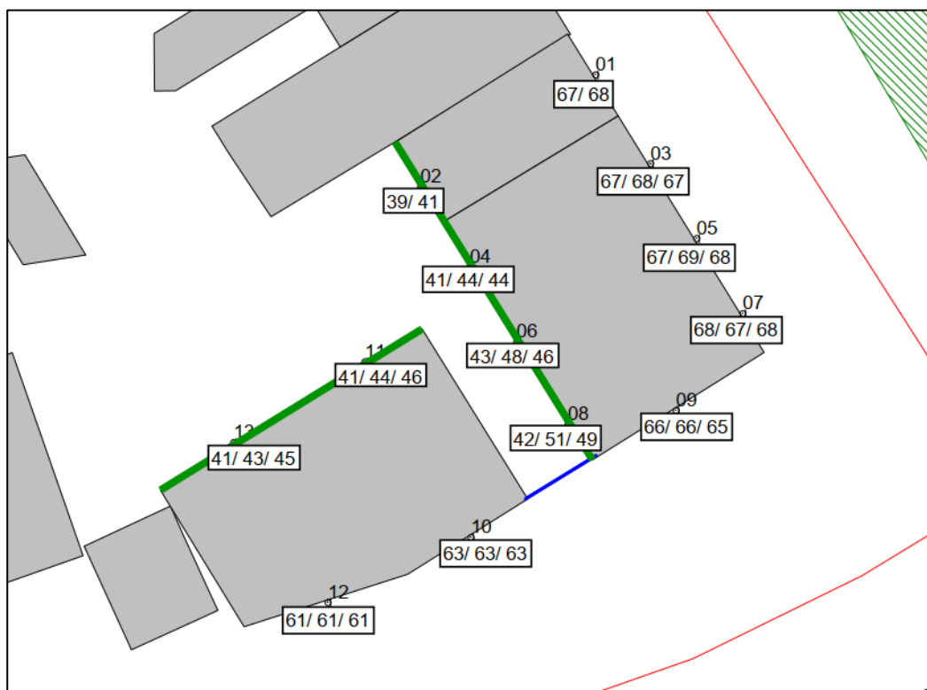
Figuur 5.4: Cumulatieve geluidbelasting incl. 30 km/uur wegen op de nieuwbouw excl. aftrek art. 110g Wgh (na toepassen gebouwgebonden schermen)
