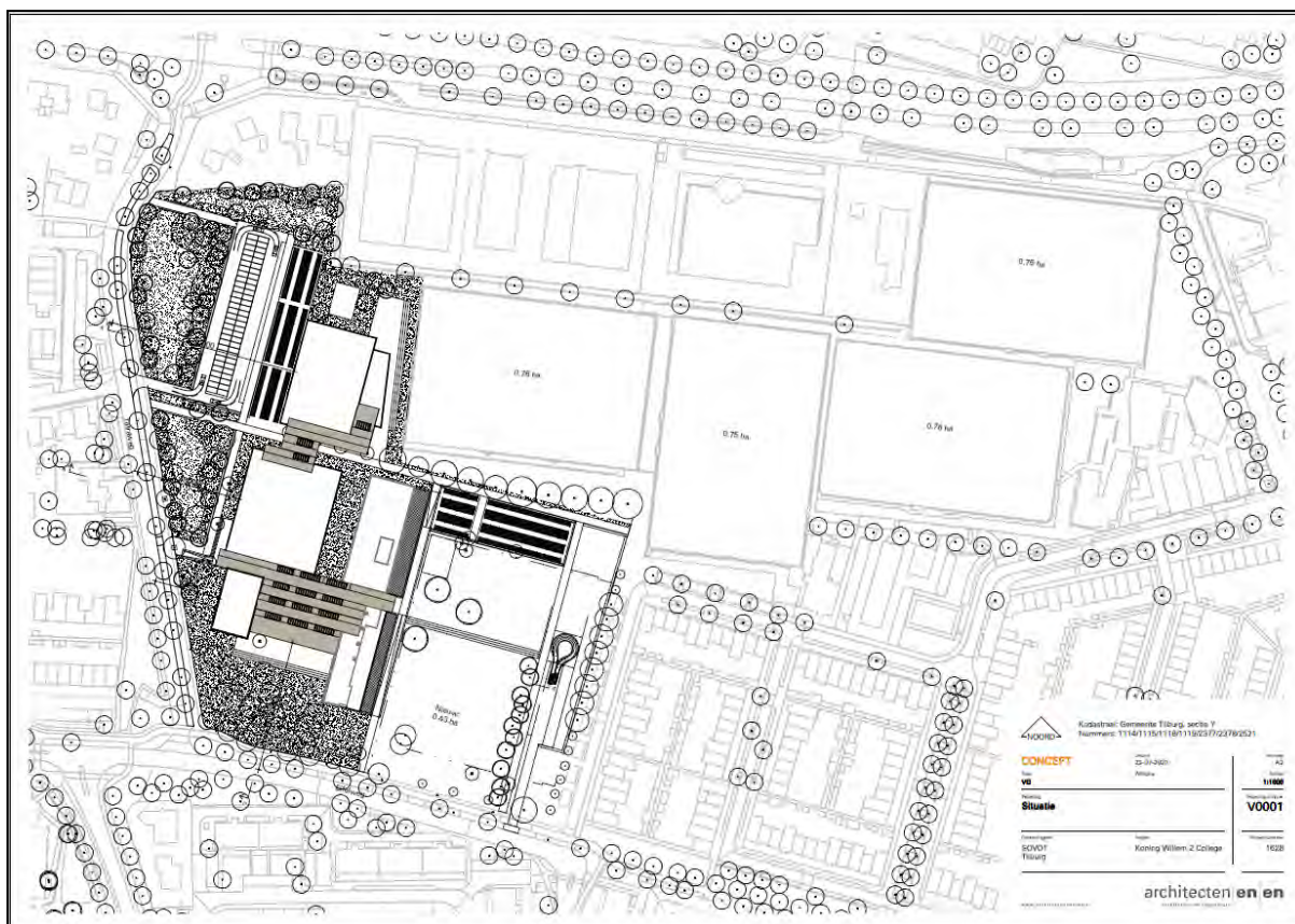
Figuur 12. Toekomstige situatie op de onderzoekslocatie (tekeningnummer V0001, d.d. 22-07-2020).
