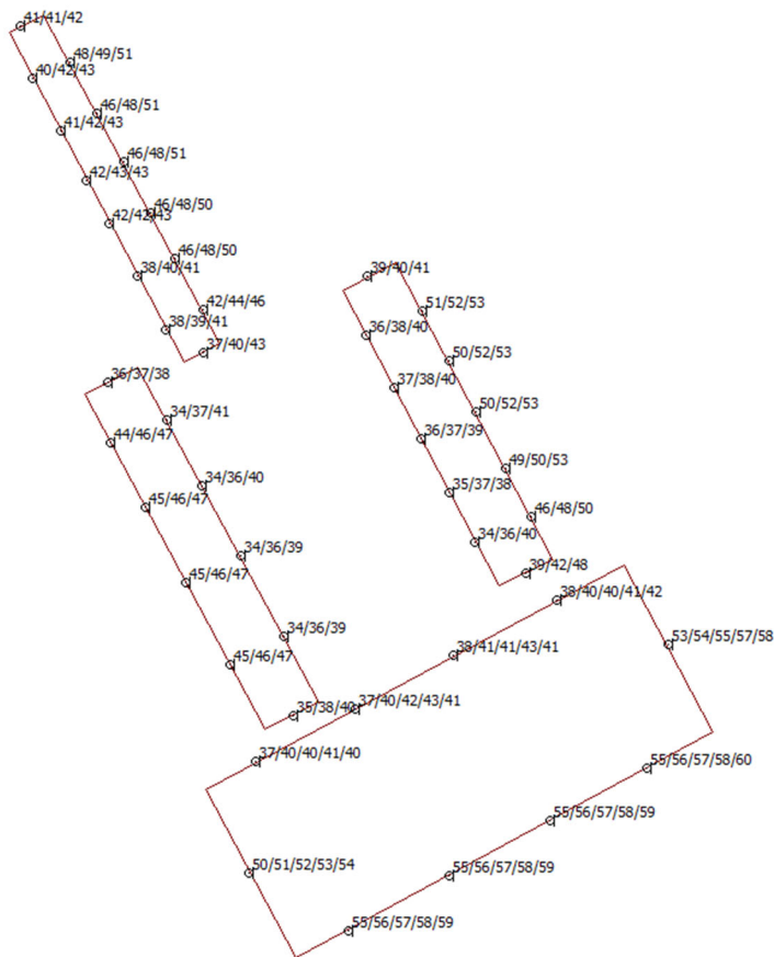
Figuur 3.2: Rekenresultaten t.g.v. railverkeer op spoorlijn Tilburg – 's-Hertogenbosch ter hoogte van het middelste bouwblok, blok 6 t/m 9
