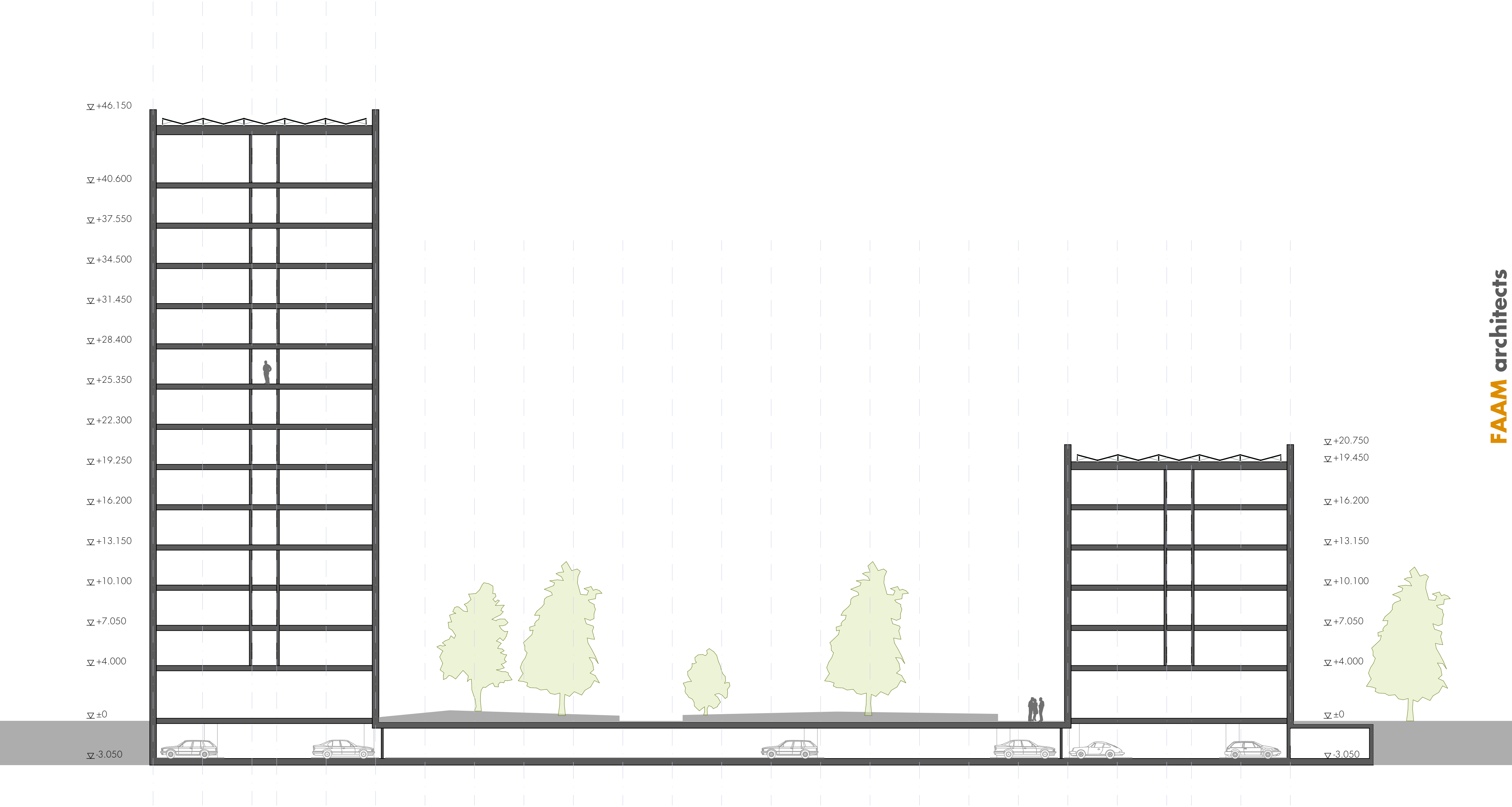
Doorsnede BB
