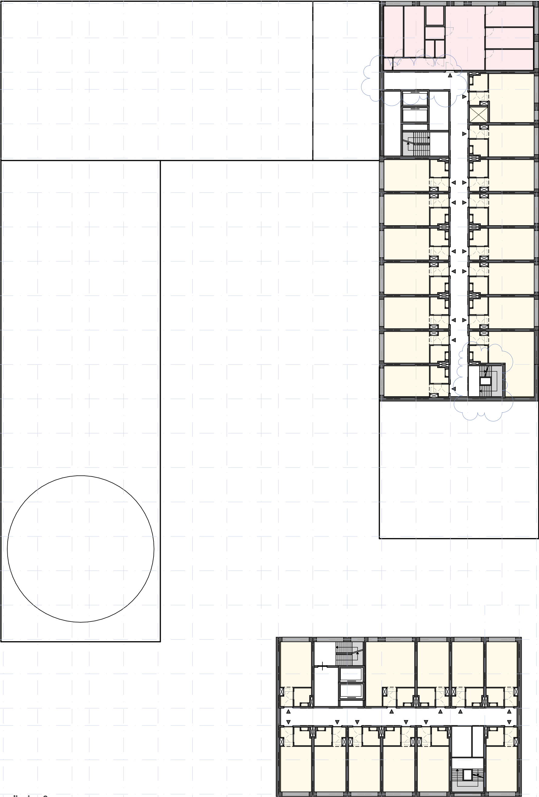
vedieping 8
