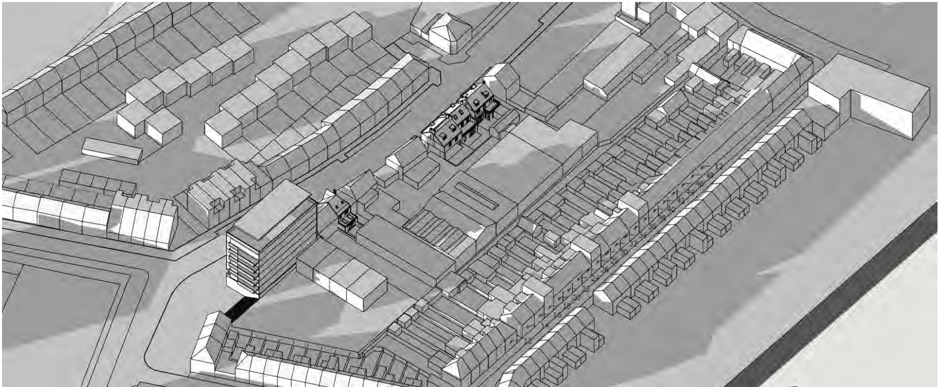
De Mersjant – zonnestudie – huidige situatie : periode 12 december om 09.00 uur
