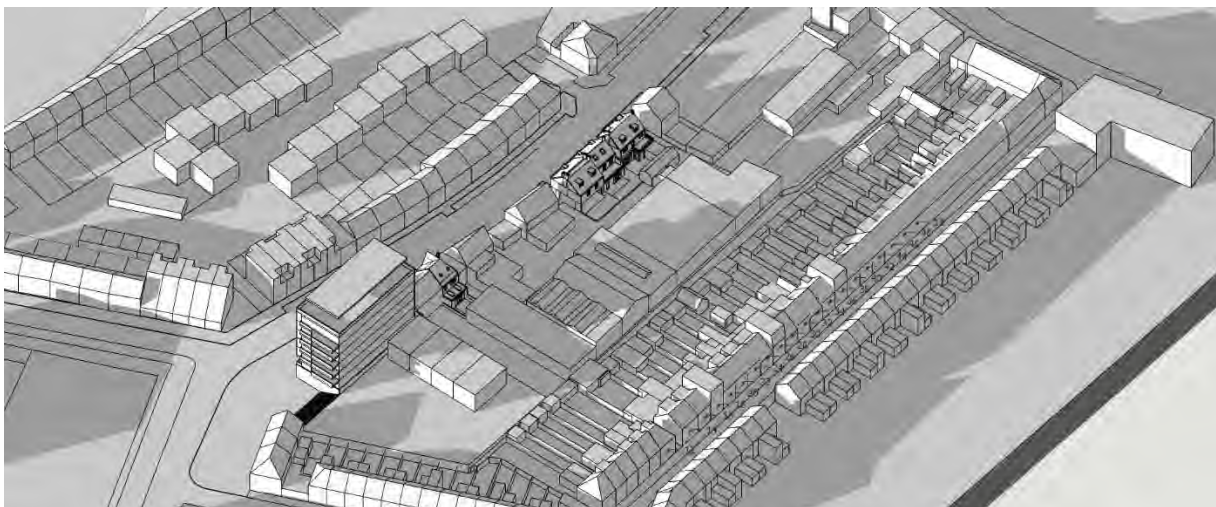
De Mersjant – zonnestudie – huidige situatie : periode 21 maart om 09.00 uur
