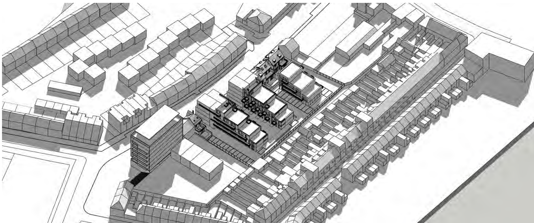
De Mersjant – zonnestudie – nieuwe stuatie met realisatie De Mersjant : periode 21 juni om 16.00 uur
