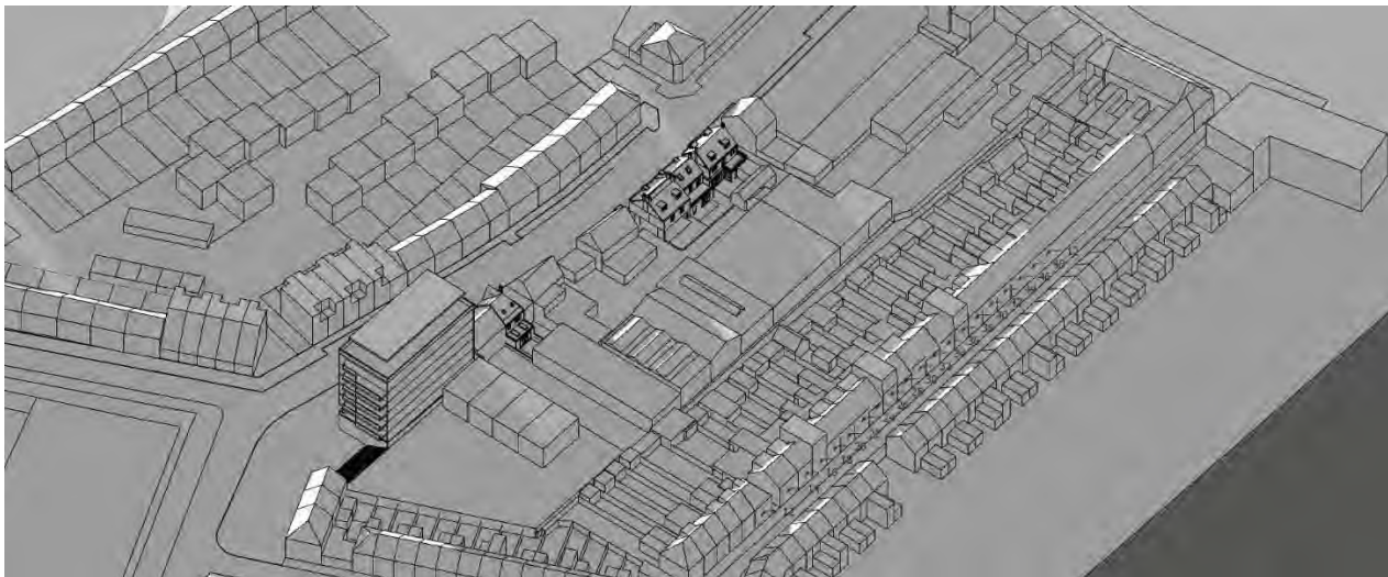
De Mersjant – zonnestudie – huidige situatie : periode 12 december om 15.00 uur
