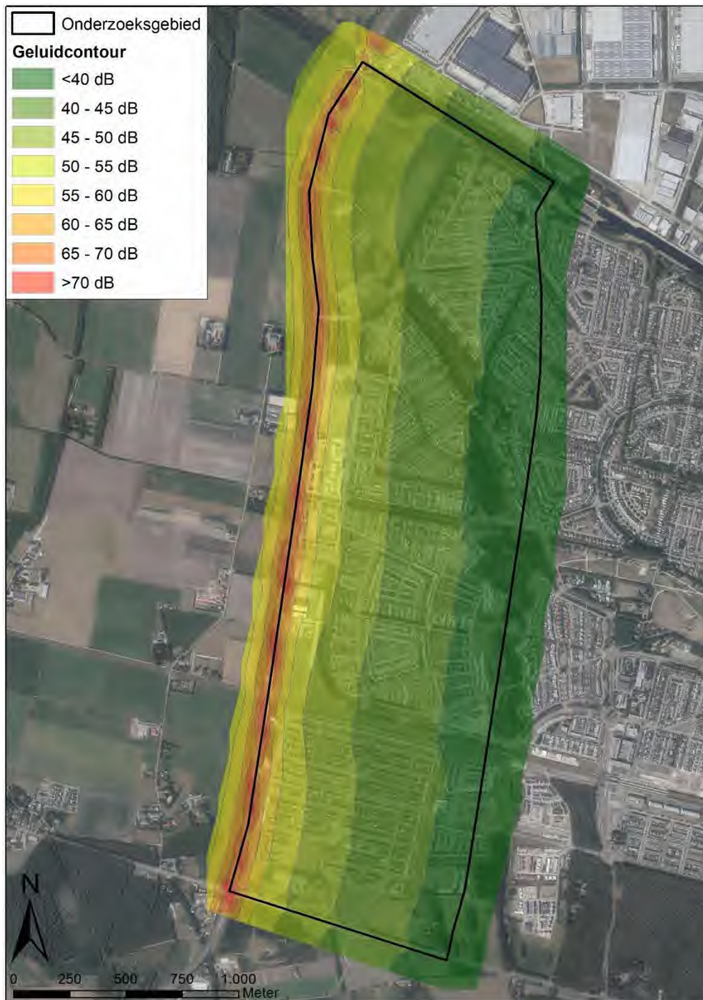
Figuur 3-1 Geluidcontouren van de huidige situatie
