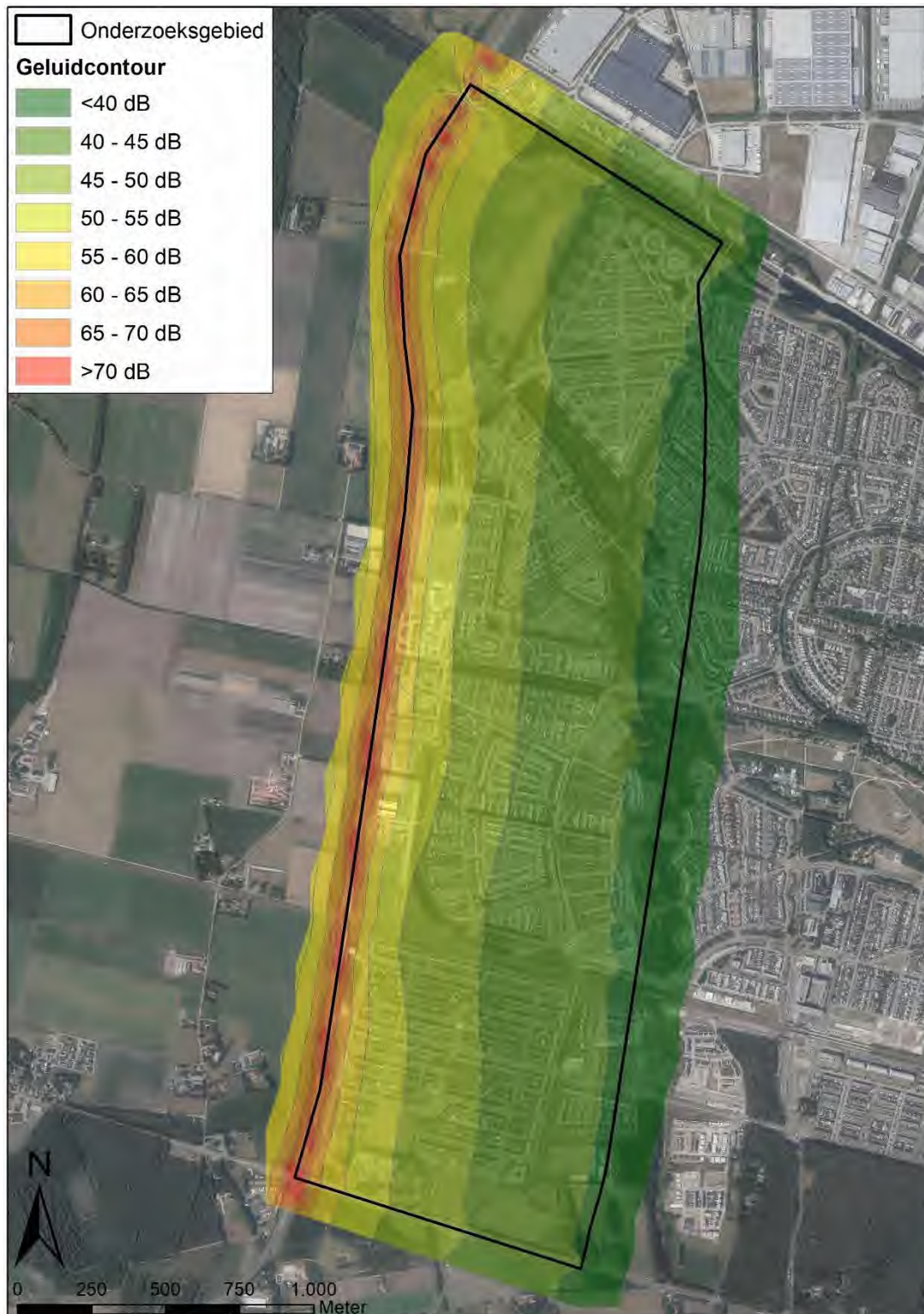
Figuur 3-3 Geluidcontouren van de plansituatie
