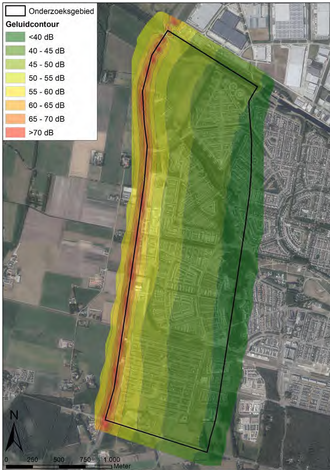
Figuur 3-2 Geluidcontouren van de autonome situatie
