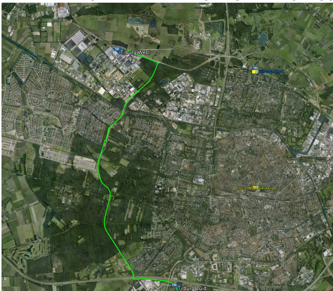
Afbeelding 1 Situatie 150kV kabelverbinding Tilburg West – Tilburg Zuid
