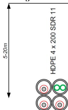
Afbeelding 3: Doorsnede HDD-boring
