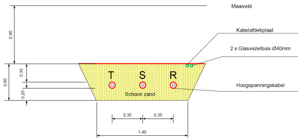
Afbeelding 1: Doorsnede openontgraving A-A
