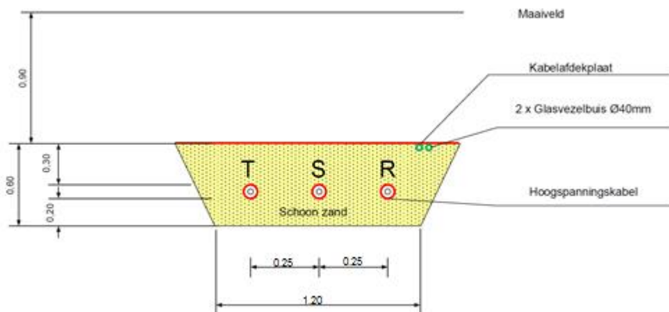
Afbeelding 2: Doorsnede openontgraving B-B
