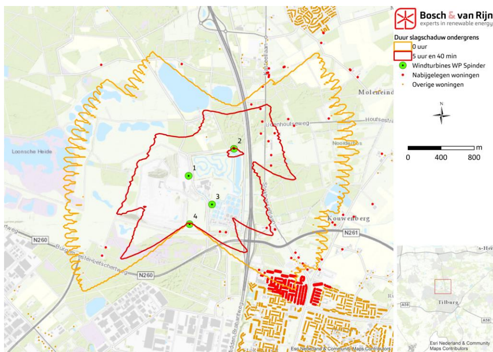
Figuur 3 – 5:40u en 0:00u slagschaduwcontour van de ondergrens. Hierbij zijn ook woningen van derden weergegevens. Dit zijn immers de objecten waarvoor de norm geldt. (Er liggen geen andere gevoelige objecten, zoals scholen en ziekenhuizen, binnen en nabij de contour).
