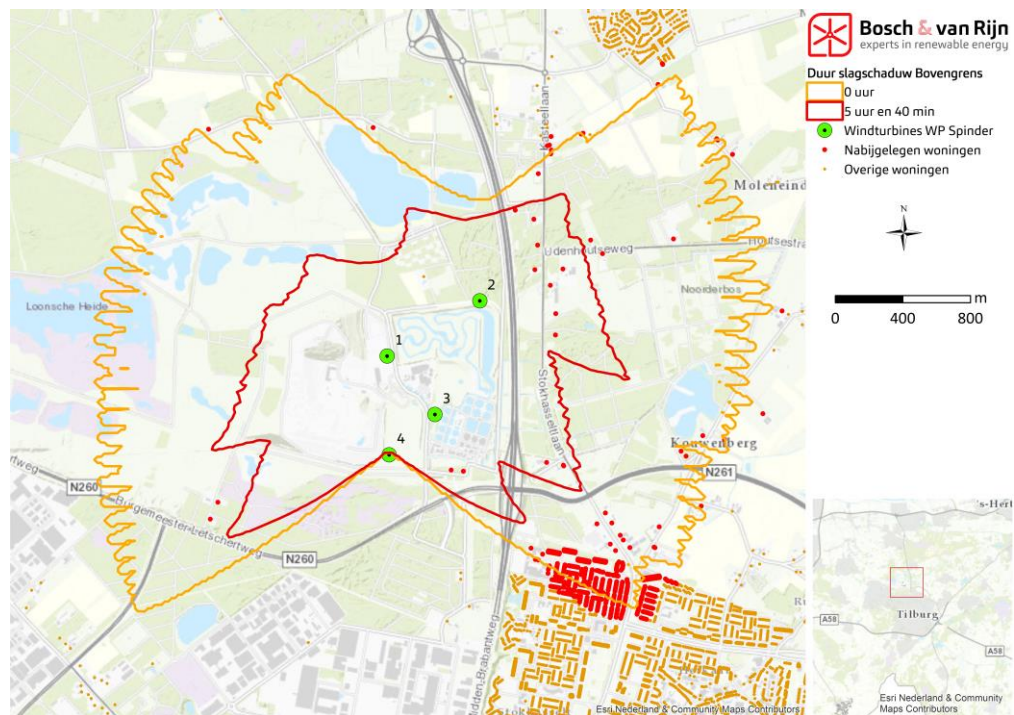
Figuur 4 – 5:40u en 0:00u slagschaduwcontour van de bovengrens. Hierbij zijn ook woningen van derden weergegeven. Dit zijn immers de objecten waarvoor de norm geldt. (Er liggen geen andere gevoelige objecten, zoals scholen en ziekenhuizen, binnen en nabij de contour).
