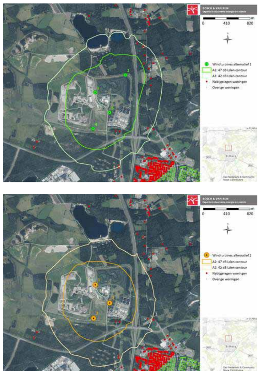
Figuur 11.2 Belasting met geluid van de omgeving door alternatief 4 turbines en alternatief 3 turbines (42 en 47 dB(A)-contour).
