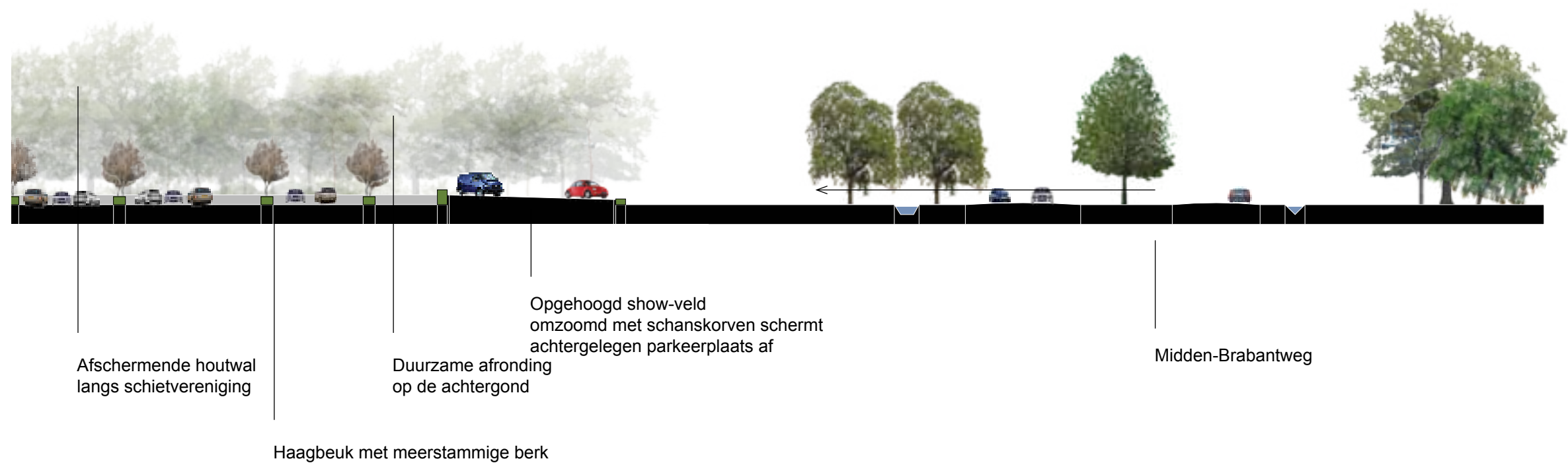
Doorsnede a-a'
