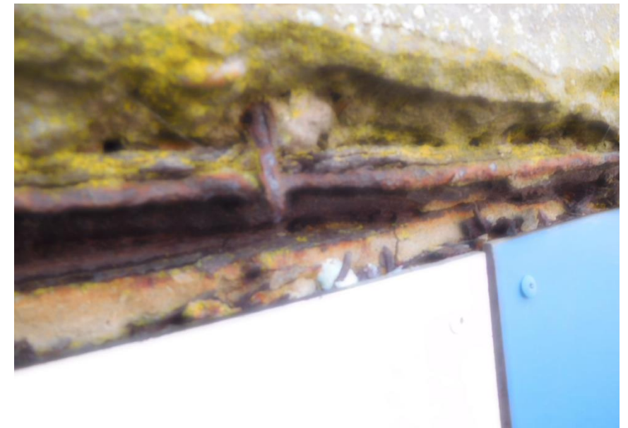
Figuur 15: Niet doorlopende kier boven trespaplaten bij afgetimmerde deur aan de Westgroeneweg
