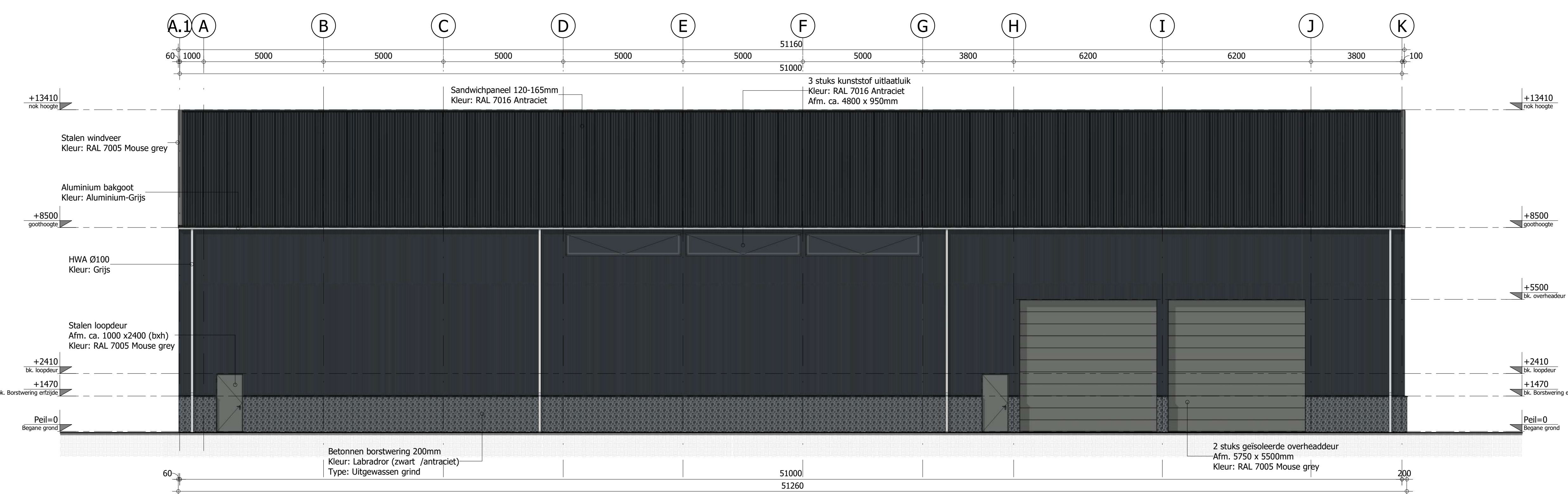
Voorgevel AS-1
