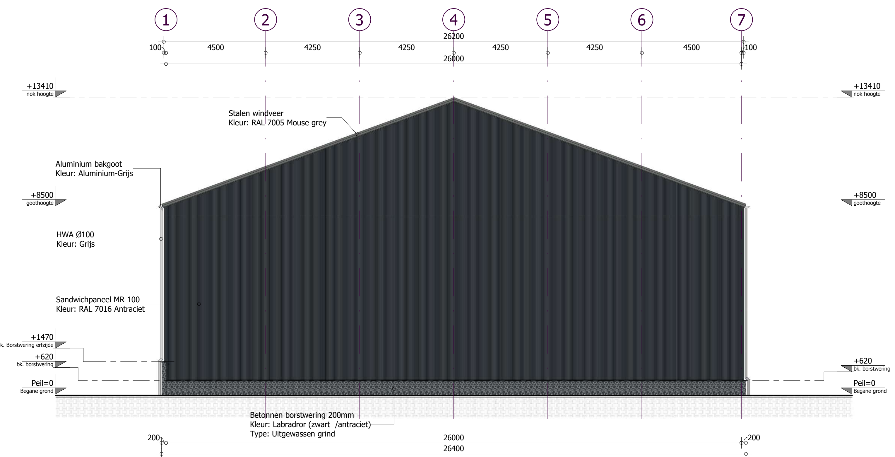
Rechter zijgevel AS-K
