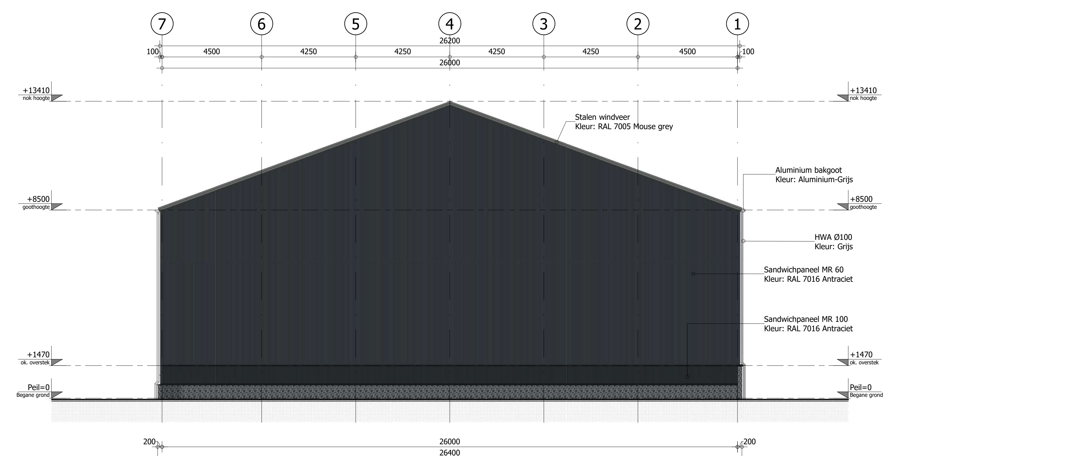
Linker zijgevel AS-A.1
