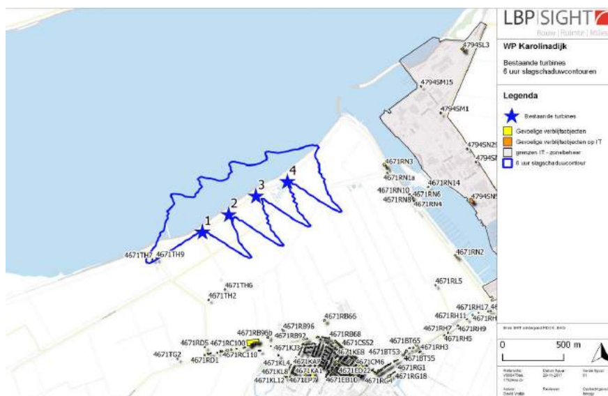
Figuur 4.3 6 uur slagschaduwcontour huidige windpark
