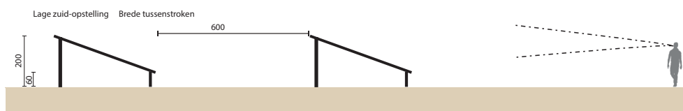
Hoge en lage zuid opstelling met smalle en brede tussenstroken
