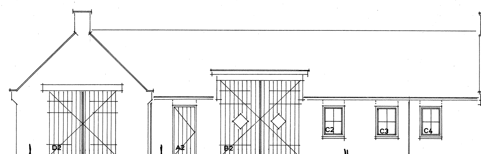
NOORDWESTGEVEL
