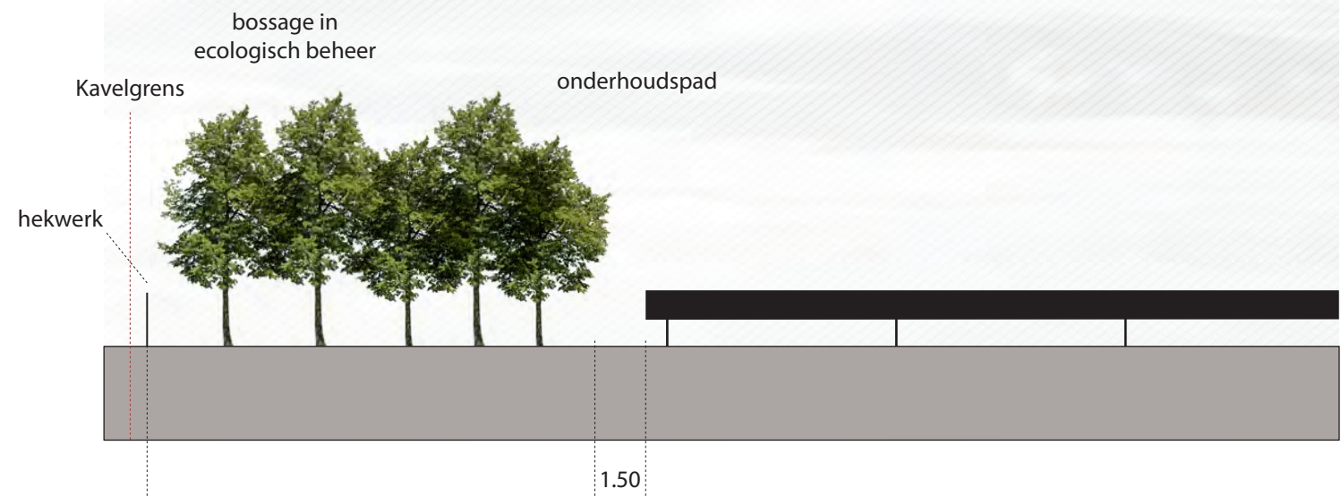
Doorsnede B
