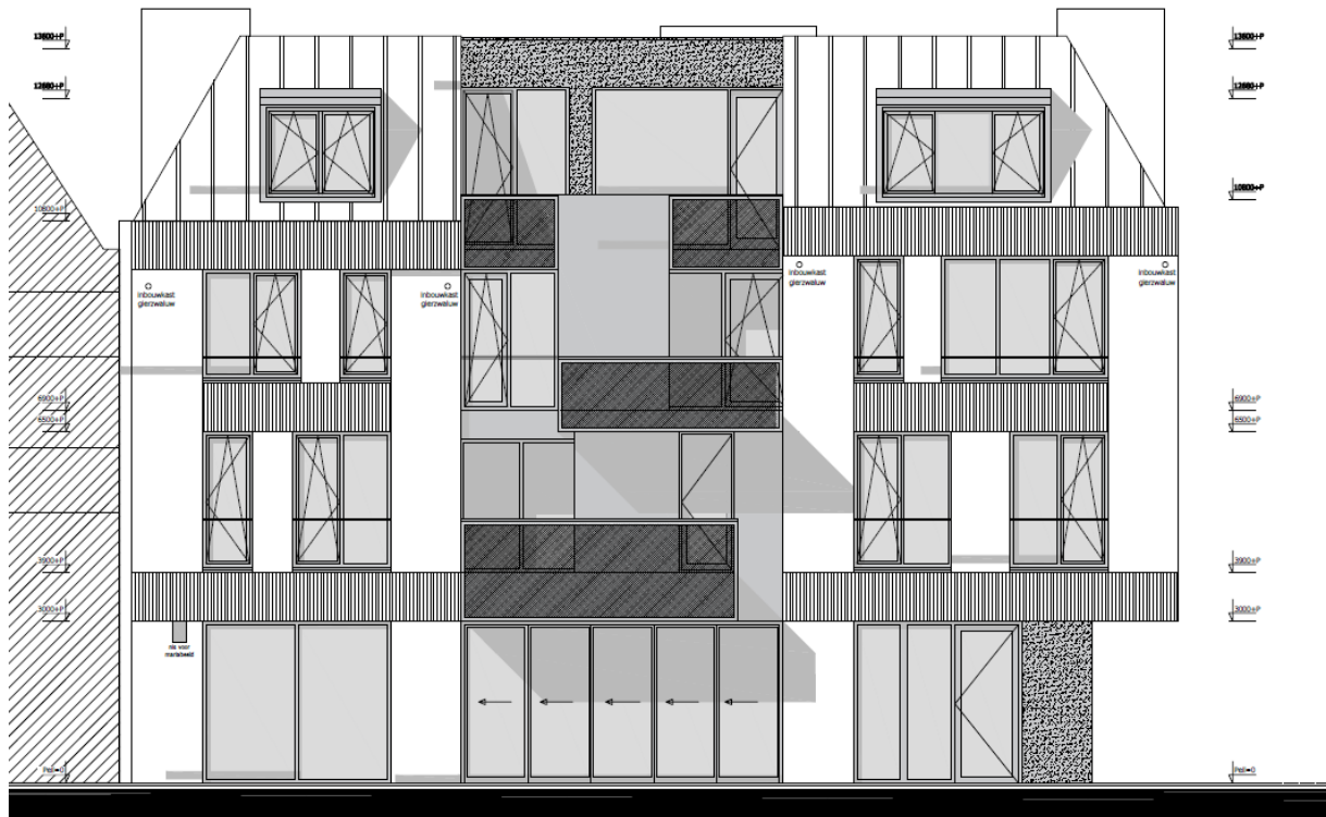
Voorgevel
