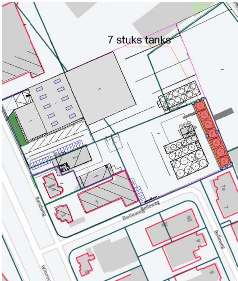
Afbeelding 8. Situering bouwvlak.
