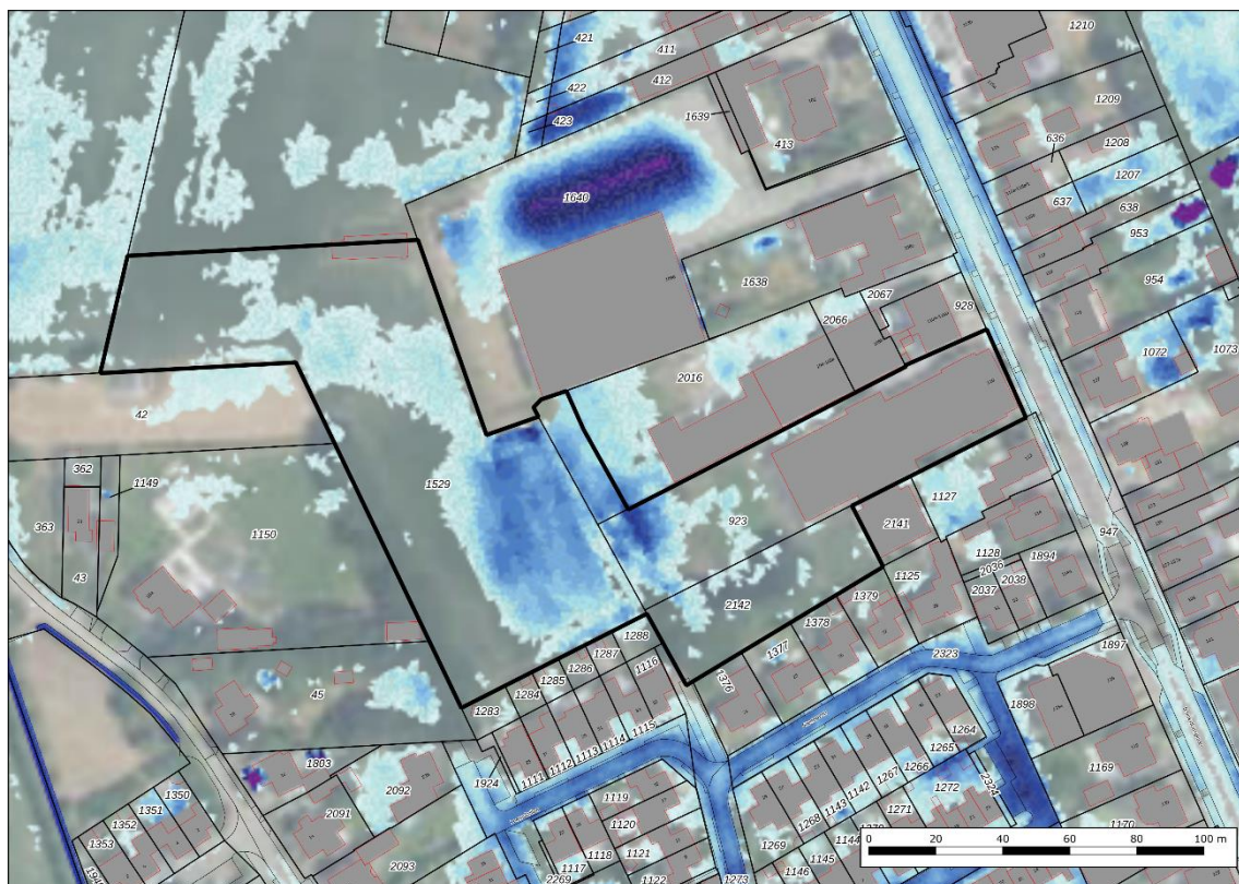
Figuur 4.4 Stresstest, bui 160 mm in 2 uur
