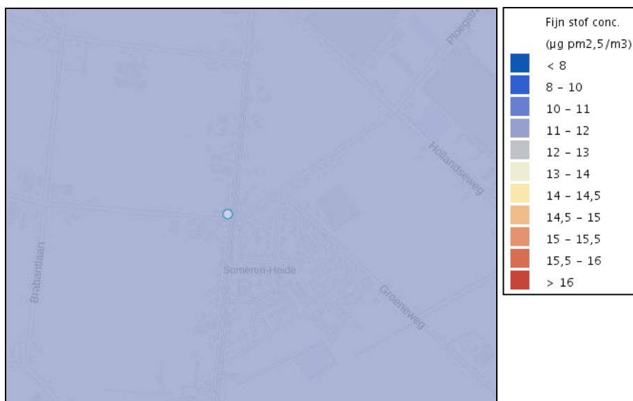
Figuur 9: Fijnstof 2019 \text{PM}_{2,5} (bron: Atlas leefomgeving) voor het plangebied
