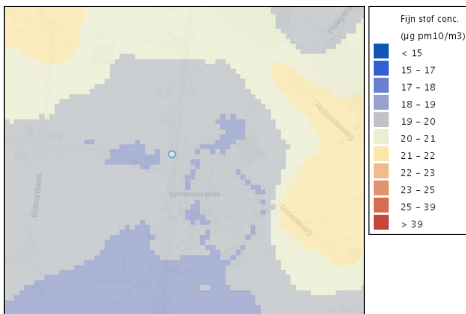
Figuur 8: Fijnstof 2019 \text{PM}_{10} (bron: Atlas leefomgeving) voor het plangebied
