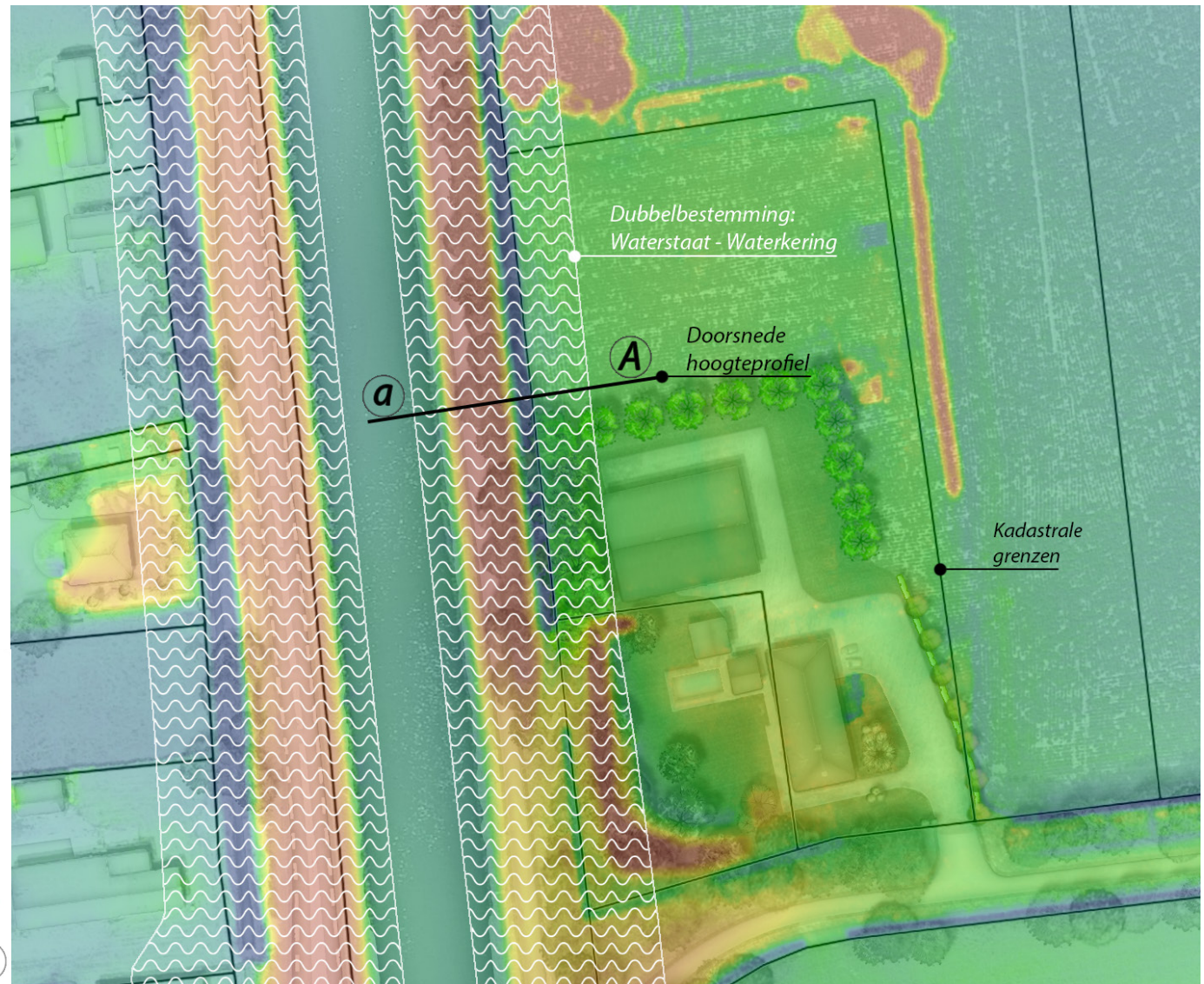
Projectie dubbelbestemming 'Waterstaat – Waterkering' op hoogtekaart & inrichtingstekening inpassing
