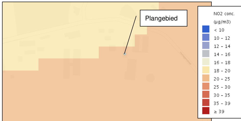
Figuur 29: Uitsnede kaart fijnstof fijnstofdioxide 2017 waarop de ligging van het plangebied is aangeduid
