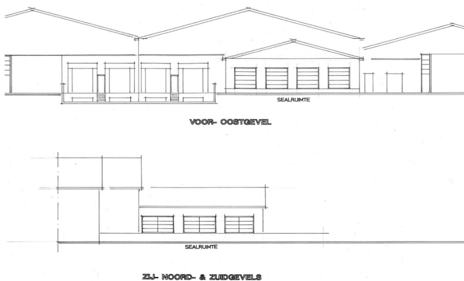
Figuur 15: Voorzijde van het bedrijf met de beoogde sealruimte en een zijaanzicht van de beoogde sealruimte
