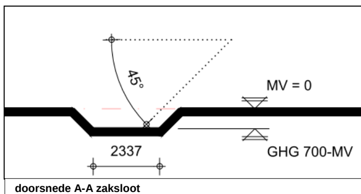
doorsnede A-A zaksloot
