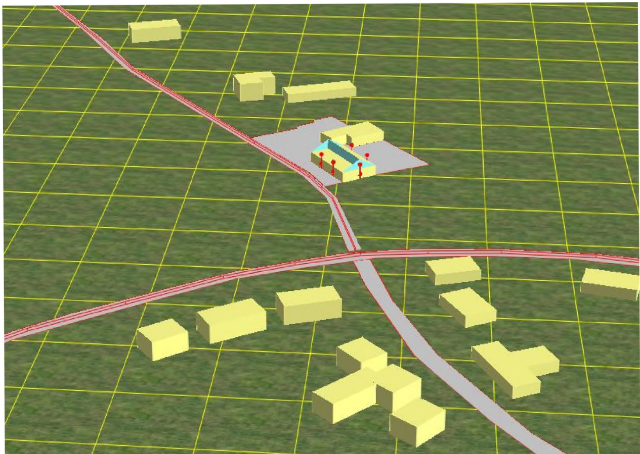
Afbeelding 2. Rekenmodel, 3d-weergave
