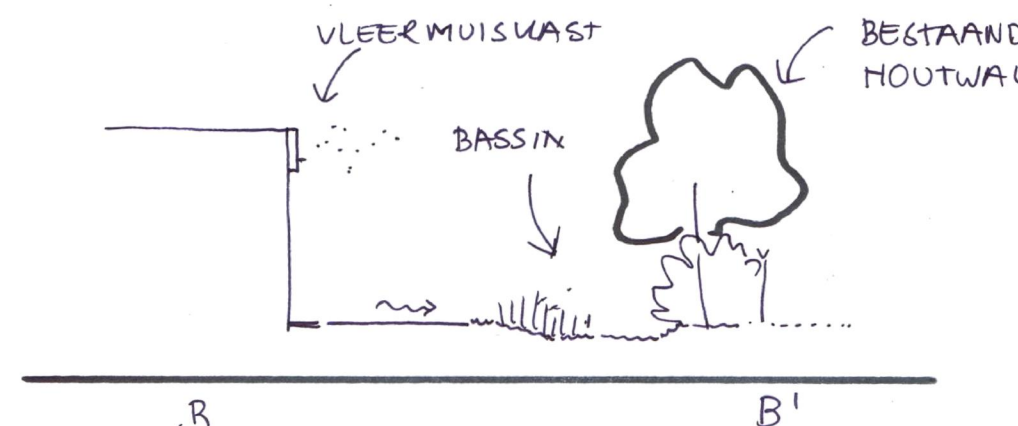
Profiel BB'
