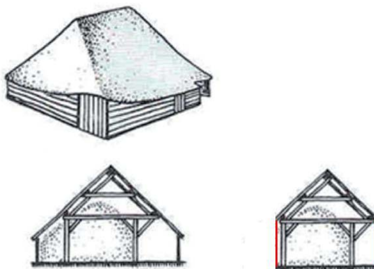
Tekening van een klassieke Vlaamse schuur (links) en (rechts) in rood de situatie bij de betreffende schuur in Schijf. Bron: Hekker 1991.
