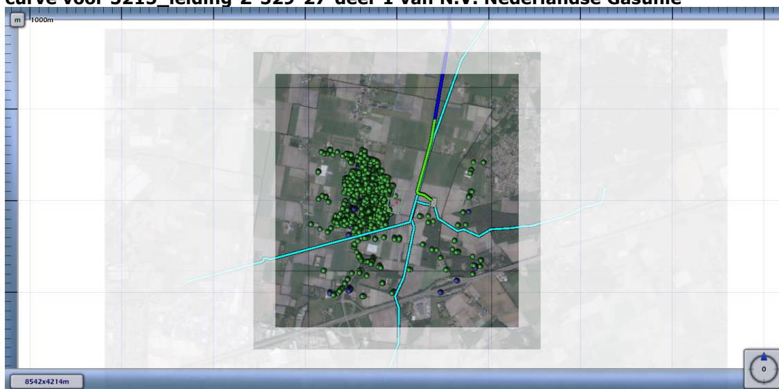
Figuur 4.5 Kilometer leiding behorende bij de maximale overschrijding van de FN-curve voor 5215_leiding-Z-529-27-deel-1 van N.V. Nederlandse Gasunie
