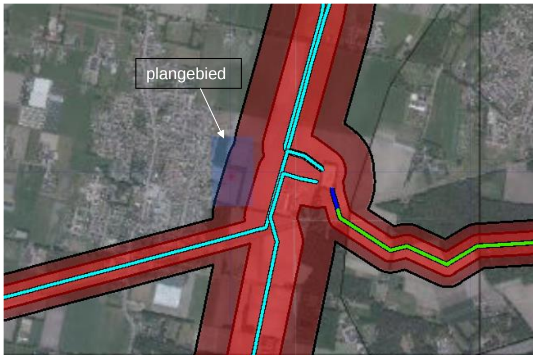
Figuur 2.1: Uitsnede CAROLA invloedsgebied buisleidingen
