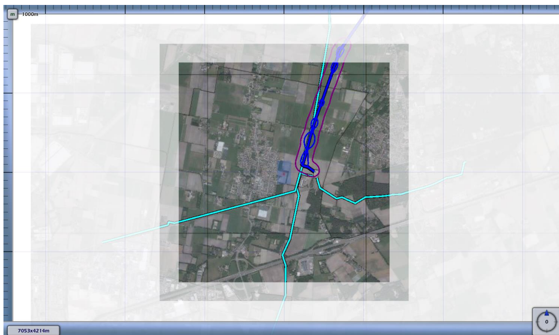
3.4 Figuur 3.4 Plaatsgebonden risico voor 5215_leiding-Z-529-26-deel-1 van N.V. Nederlandse Gasunie
