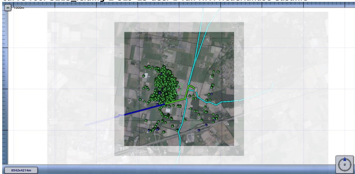
Figuur 4.3 Kilometer leiding behorende bij de maximale overschrijding van de FN-curve voor 5215_leiding-Z-529-25-deel-1 van N.V. Nederlandse Gasunie
