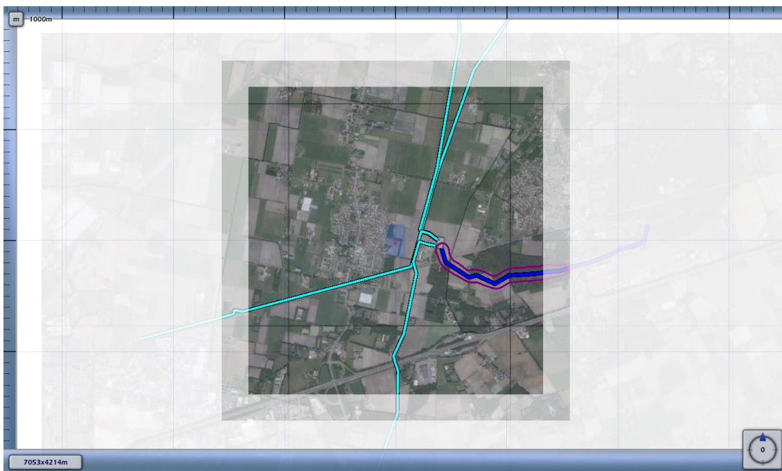
3.2 Figuur 3.2 Plaatsgebonden risico voor 5215_leiding-Z-520-36-deel-1 van N.V. Nederlandse Gasunie
