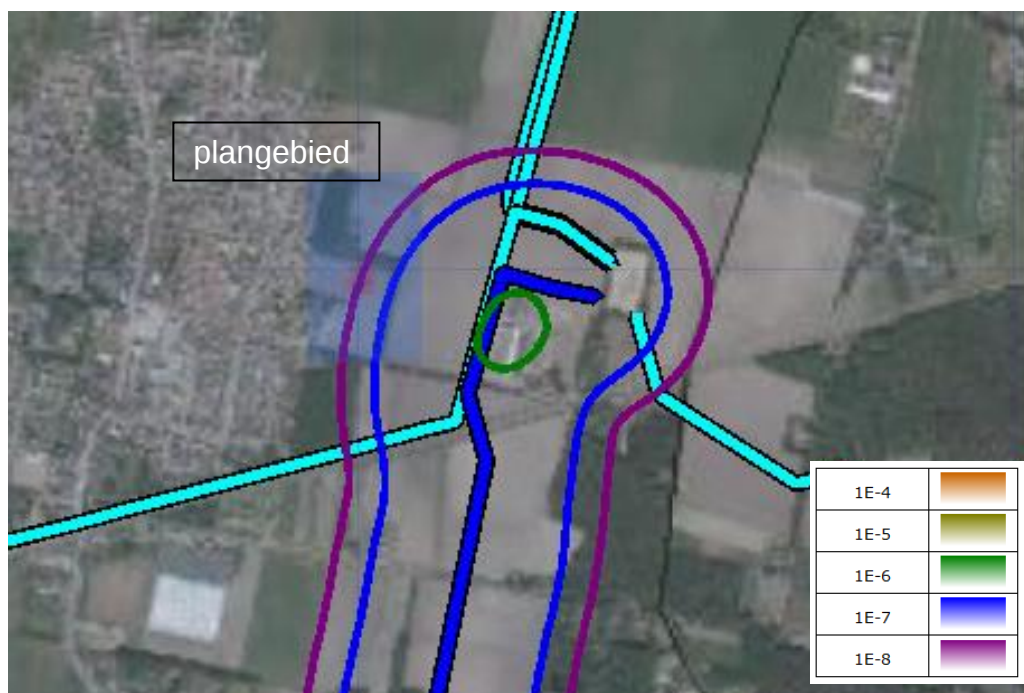
Figuur 2.2: Uitsnede CAROLA plaatsgebonden risico voor leiding A-530-03-deel-1
