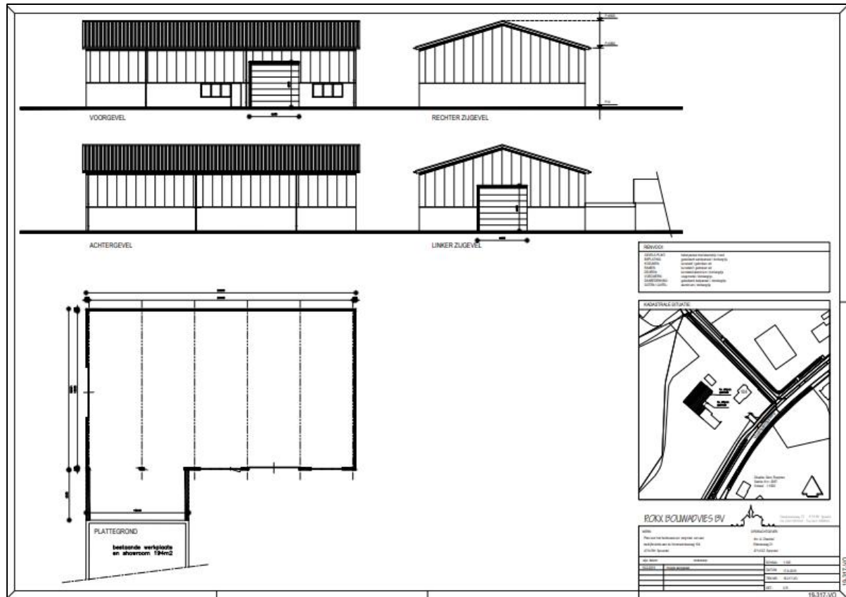
Figuur 90. Bouwplannen voor de nieuwe bedrijfsruimte. (bron: Rokx bouwadvies bv., tek.nr. 19-217-VO, 17 september 2019)
